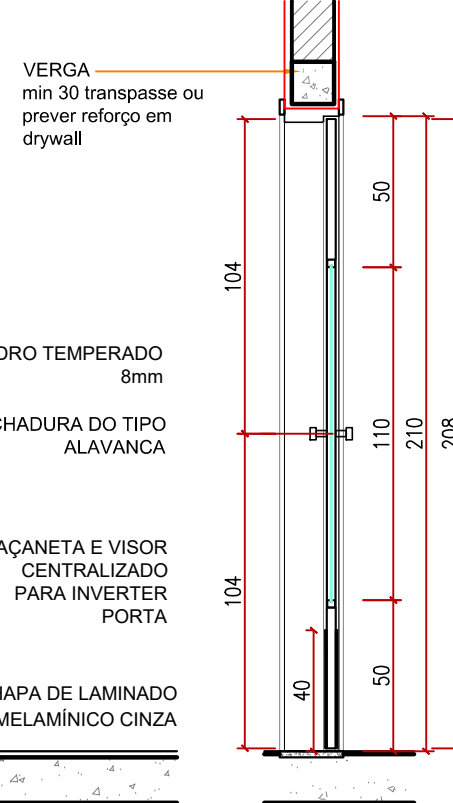
ESQUEMA DE CORTE ESC.: 1/25
