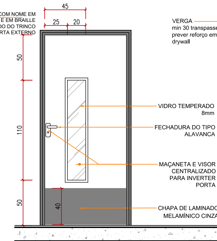
ESQUEMA VERTICAL (abertura direita – interna) ESC.: 1/25
