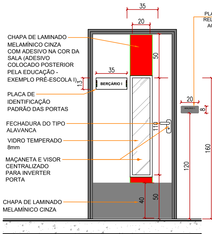
ESQUEMA VERTICAL (abertura direita – exterior) ESC.: 1/25
