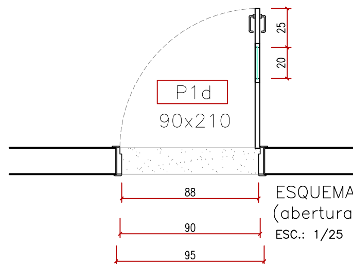
ESQUEMA VERTICAL (abertura direita – interna) ESC.: 1/25
