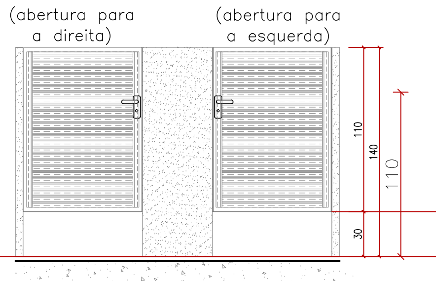
ESQUEMA VERTICAL
