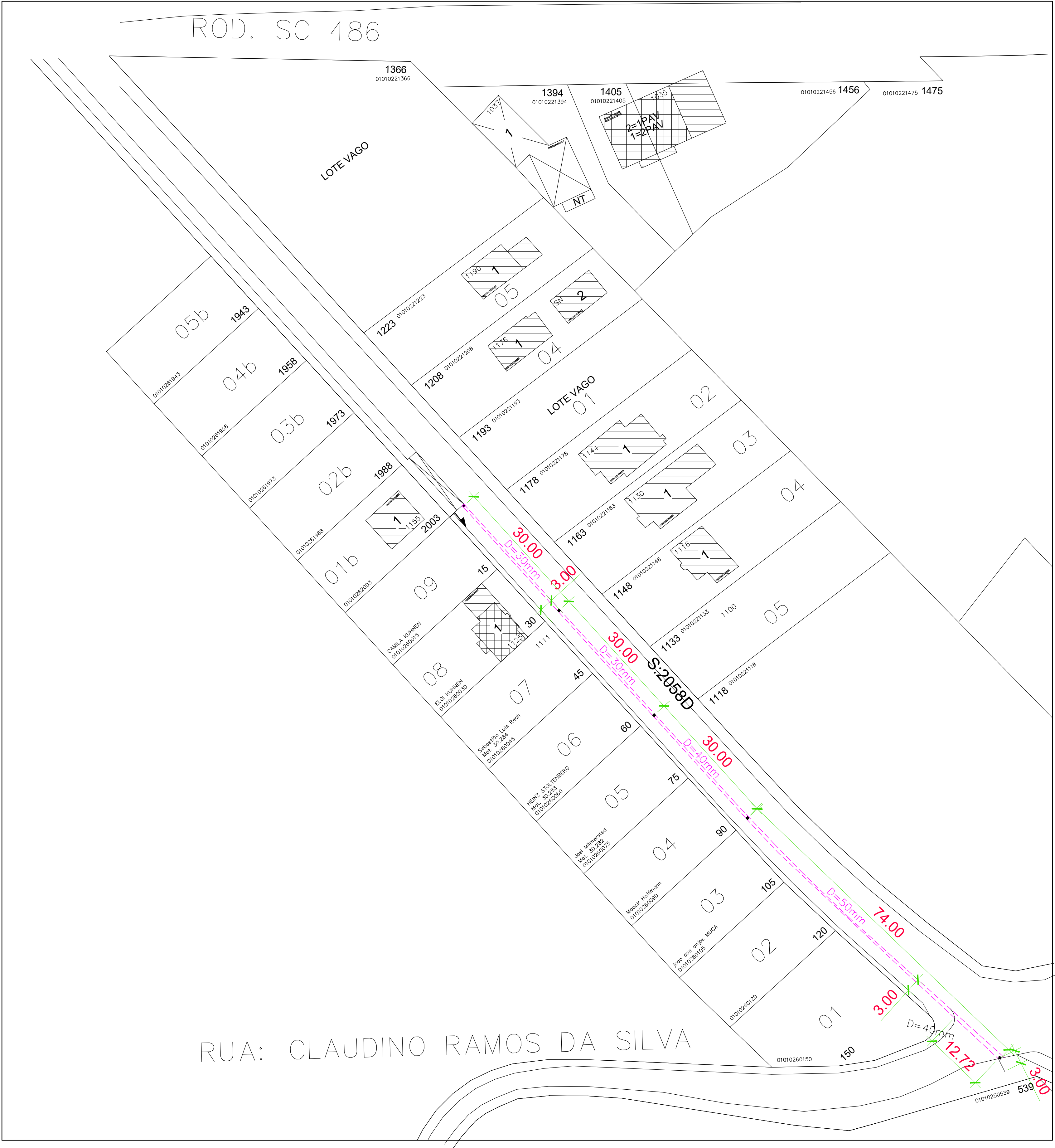
DRENAGEM - TRECHO 01 Escala_____ 1/500
