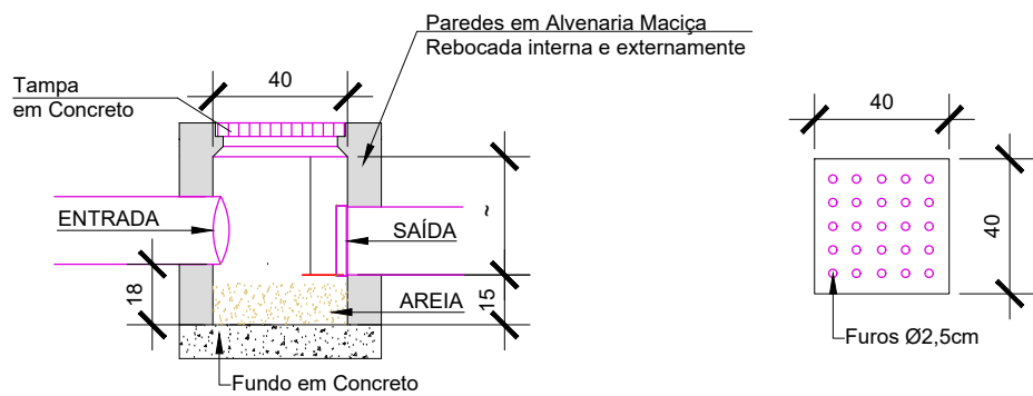
CORTE
