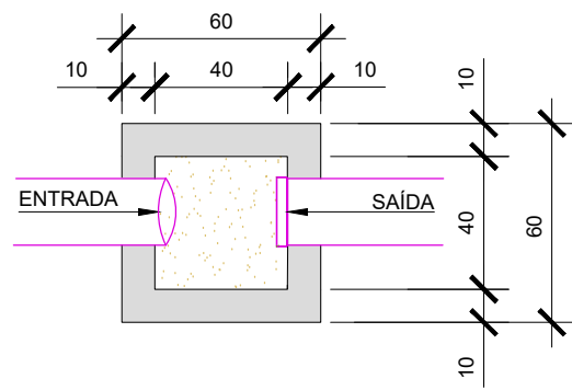
PLANTA BAIXA
