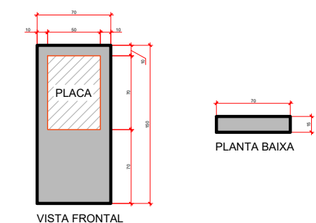
DETALHE - TOTEM DA PLACA DE INAUGURAÇÃO ESCALA: 1/50
