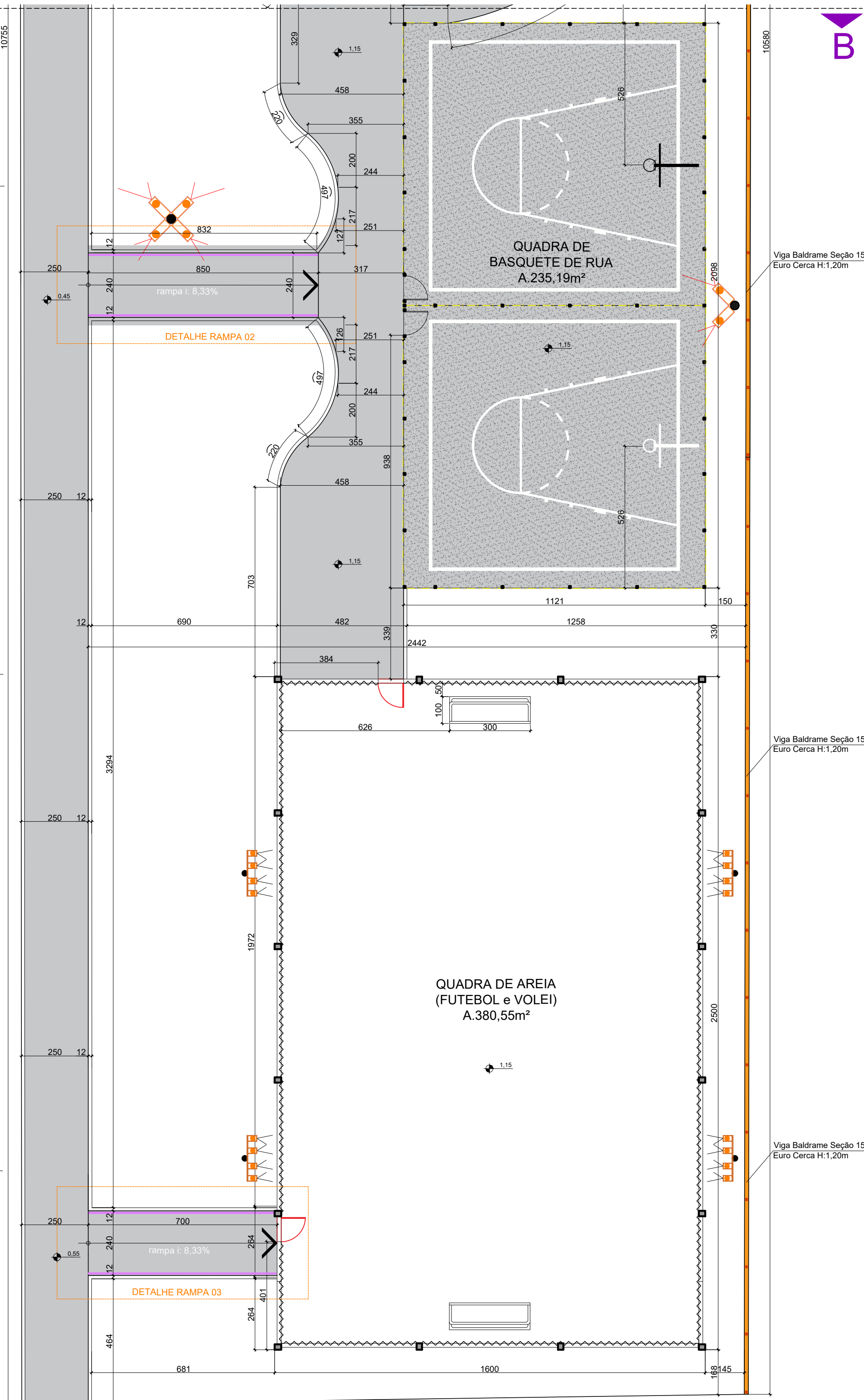
IMPLANTAÇÃO - TRECHO B ESCALA: 1/125
