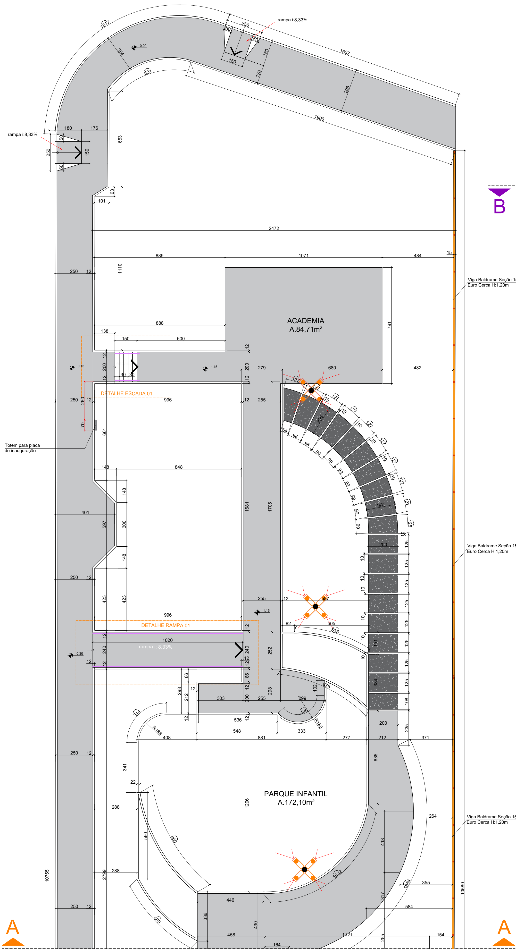
IMPLANTAÇÃO - TRECHO A ESCALA: 1/125
