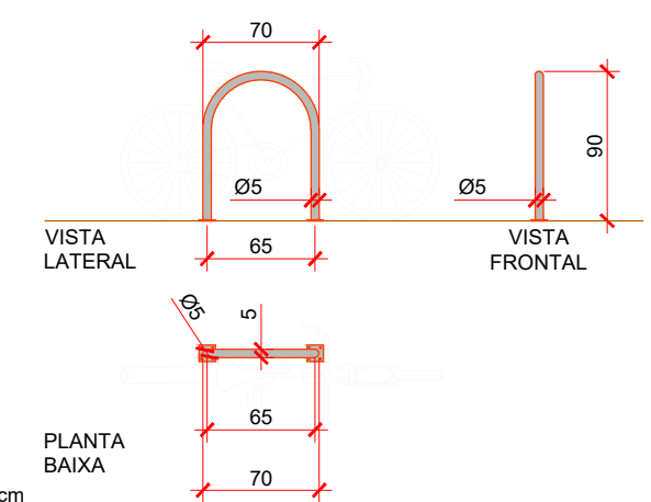
DETALHE - PARACICLO ESCALA: 1/50
