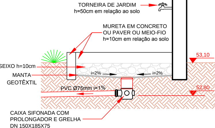
CORTE LATERAL
