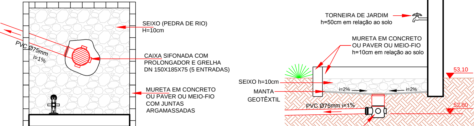
PLANTA BAIXA
