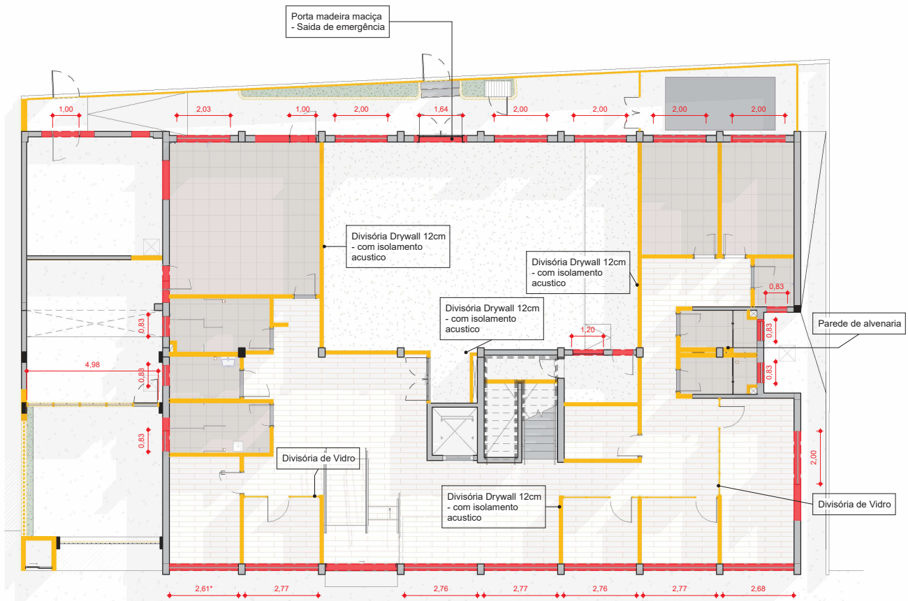
TERREO - Construção e existente 1:100
