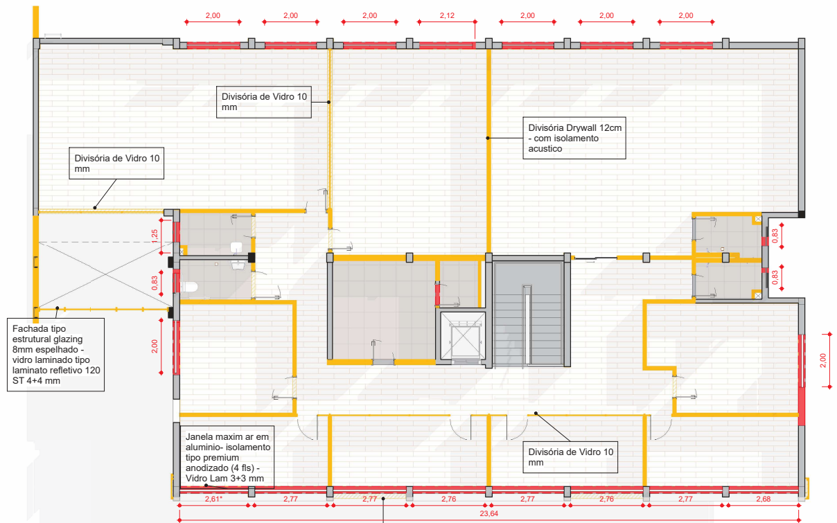
SUPERIOR - Construção e existente 1:100
