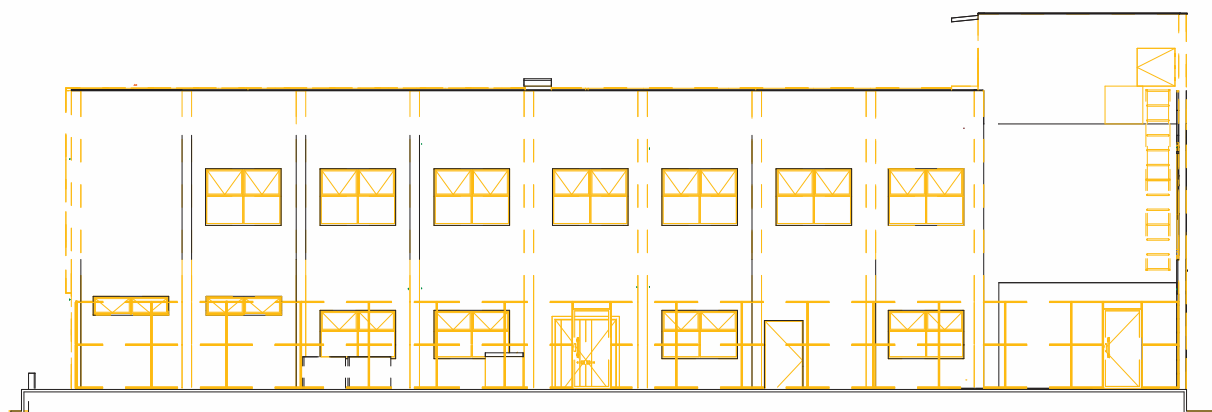
Fachada Sul - Construção 1:100
