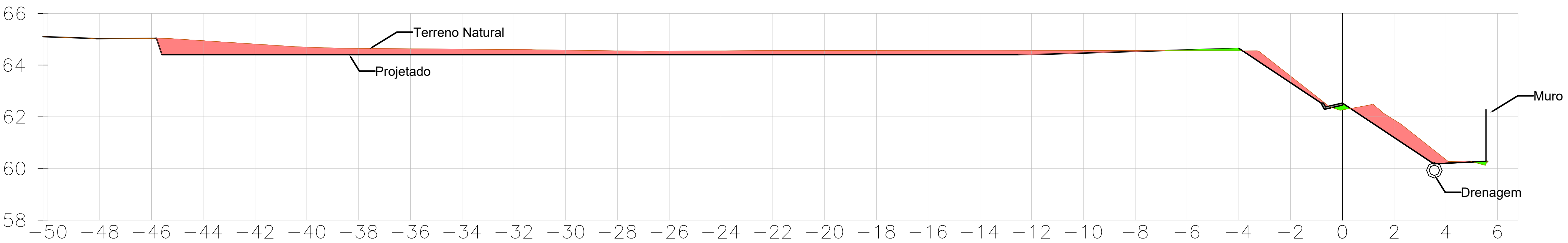
CORTE 03
