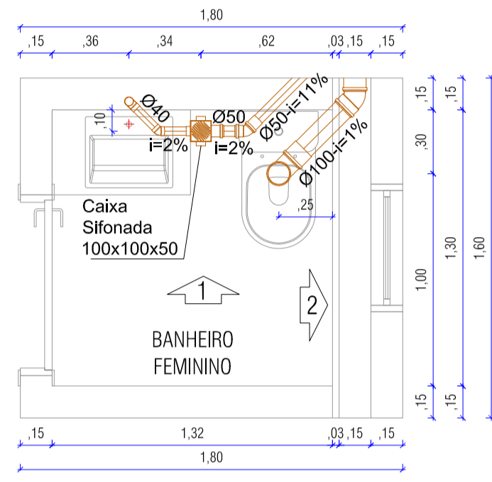
PLANTA BAIXA BANHEIRO FEMININO ESCALA 1:25
