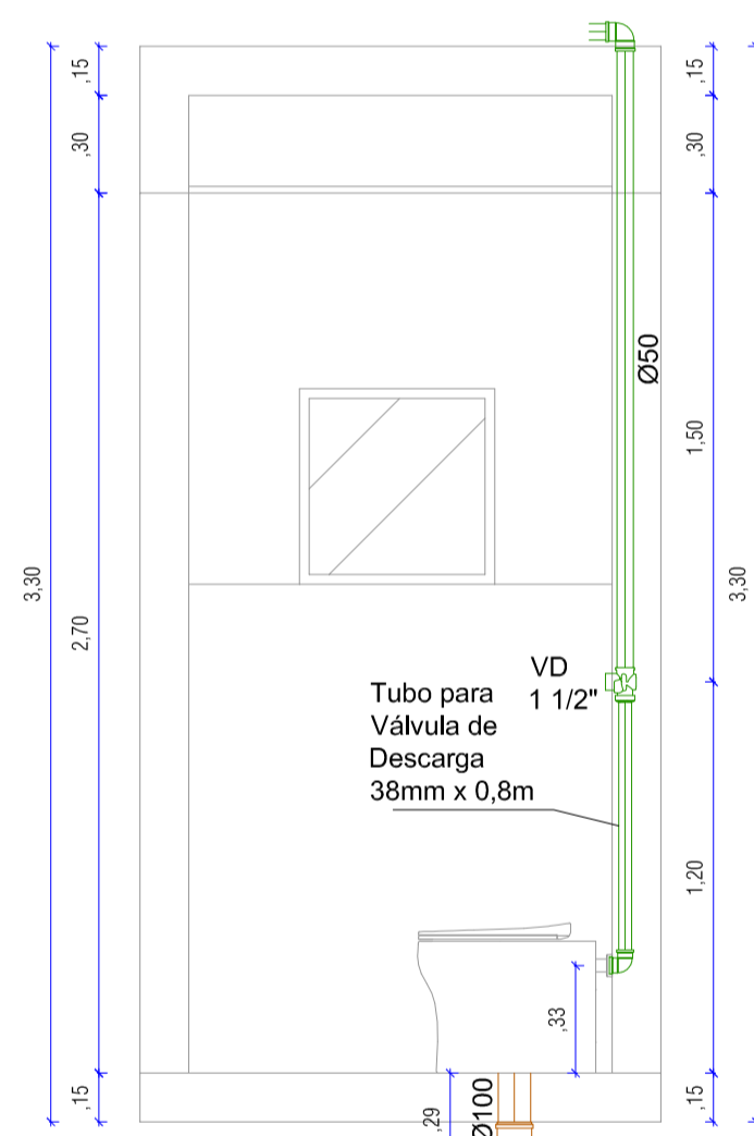
VISTA 02 ESCALA 1:25
