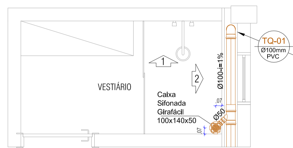
PLANTA BAIXA VESTIÁRIO ESCALA 1:25
