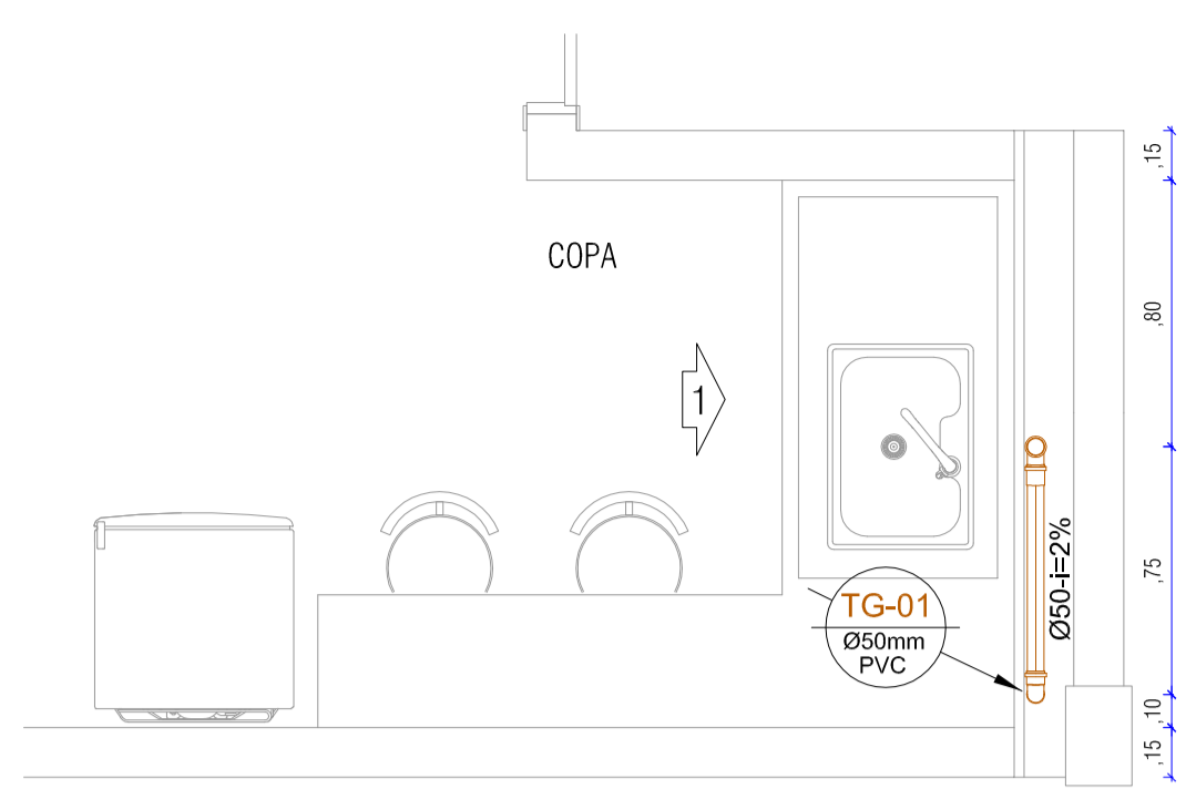
PLANTA BAIXA COPA ESCALA 1:25
