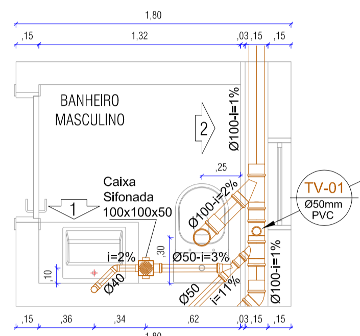
PLANTA BAIXA BANHEIRO MASCULINO ESCALA 1:25
