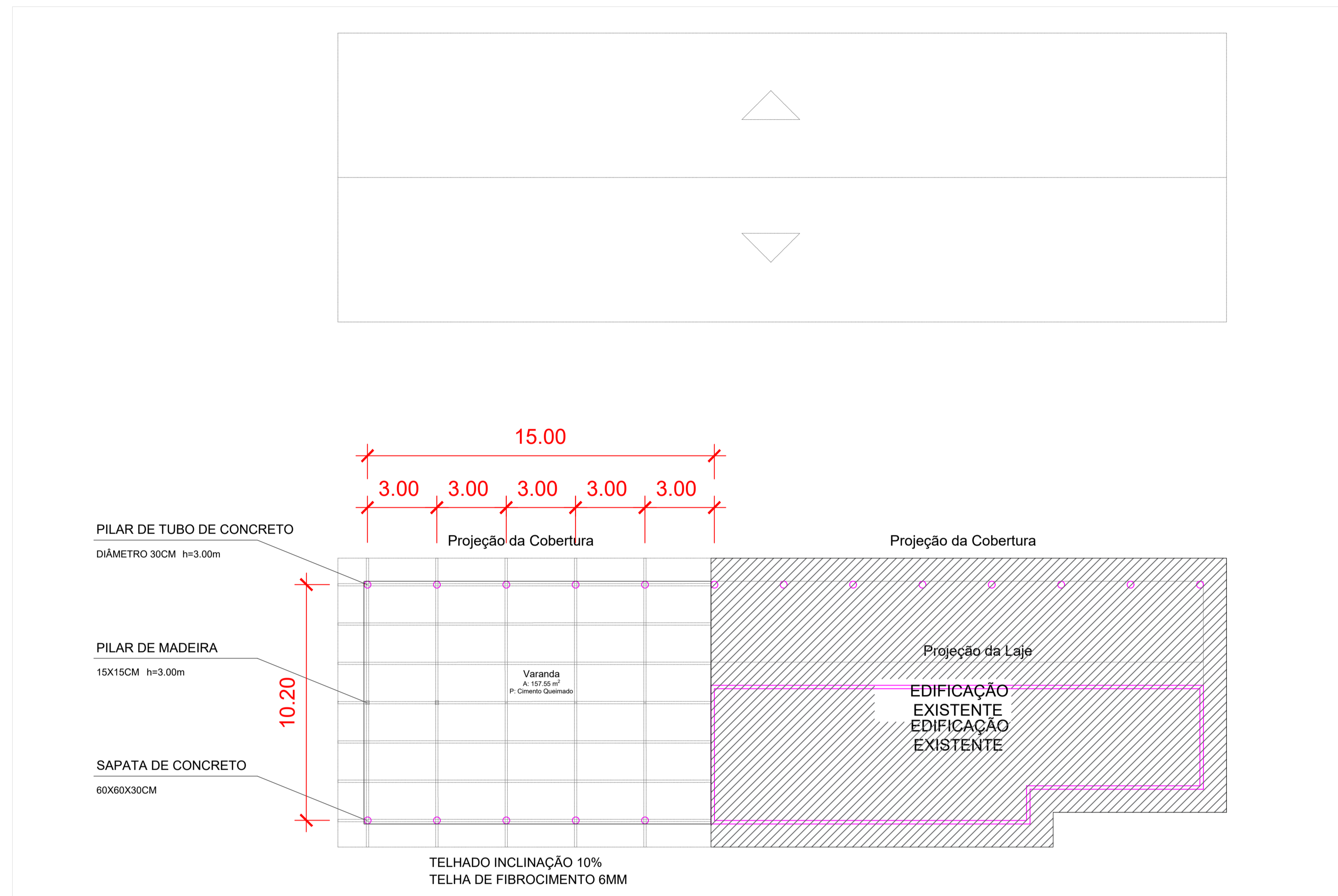
PLANTA BAIXA ÁREA AMPLIAÇÃO ESCALA 1/500
