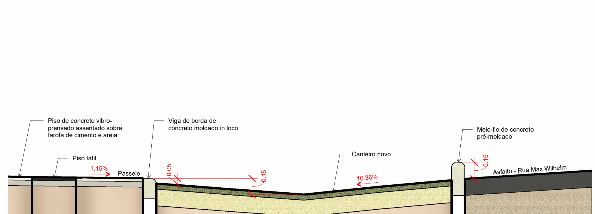
6 CORTE ESQUEMÁTICO CANTEIROS ESCALA 1:20
