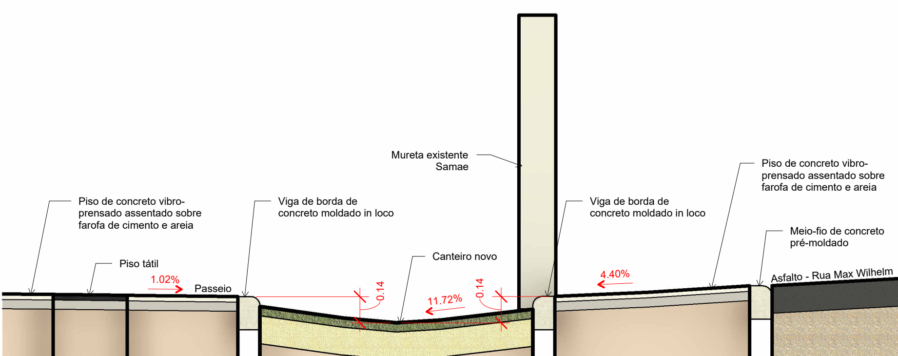
7 CORTE CANTEIRO 2 ESCALA 1:20
