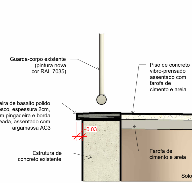
9 DETALHE SOLEIRA DE BASALTO ESCALA 1:10
