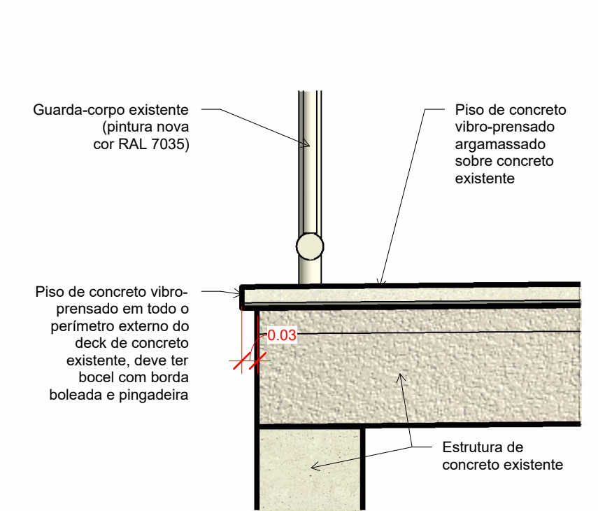
8 DETALHE PISO SOBRE CONCRETO EXISTENTE ESCALA 1:10
