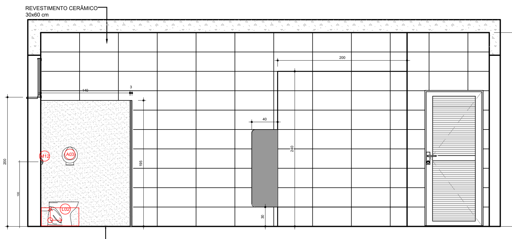
ELEVÇÃO 4 Escala 1:25
