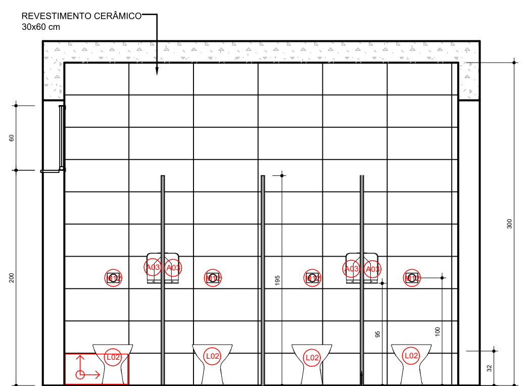
ELEVÇÃO 2 Escala 1:25
