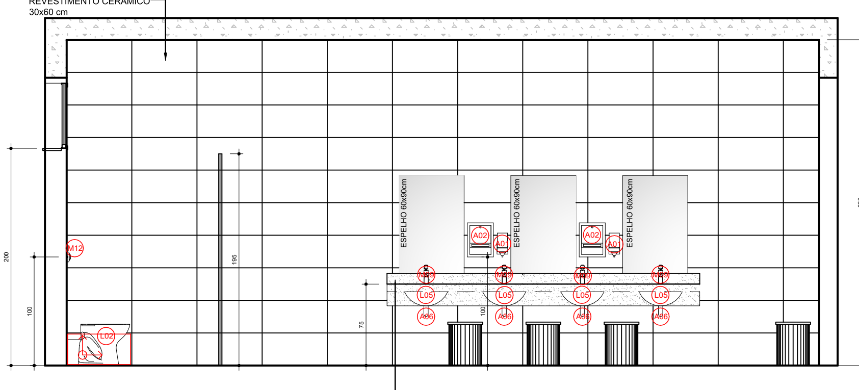
ELEVÇÃO 3 Escala 1:25
