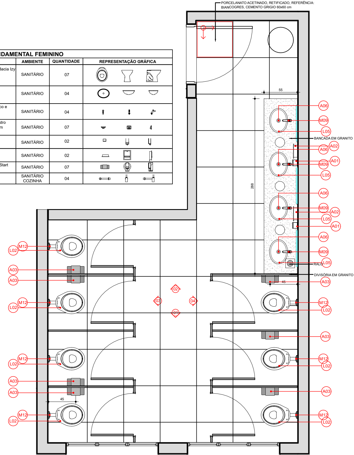
PLANTA BAIXA Escala 1:25
