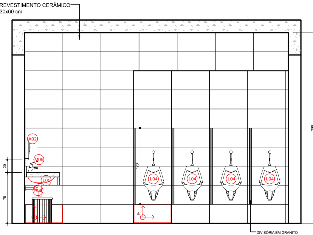
ELEVÇÃO 2 Escala 1:25
