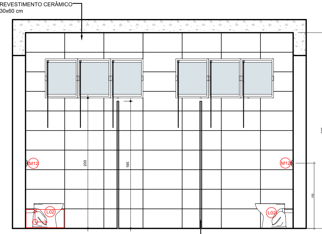
ELEVÇÃO 1 Escala 1:25
