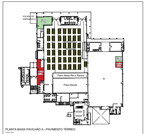
PLANTA BAIXA PAVILHÃO A - PAVIMENTO TERREO
