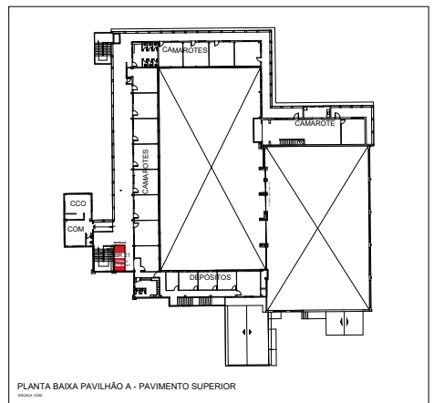
PLANTA BAIXA PAVILHÃO A - PAVIMENTO SUPERIOR
