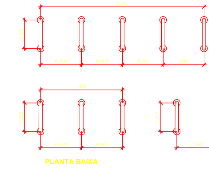
DETALHE PARACICLOS ESCALA 1:50
