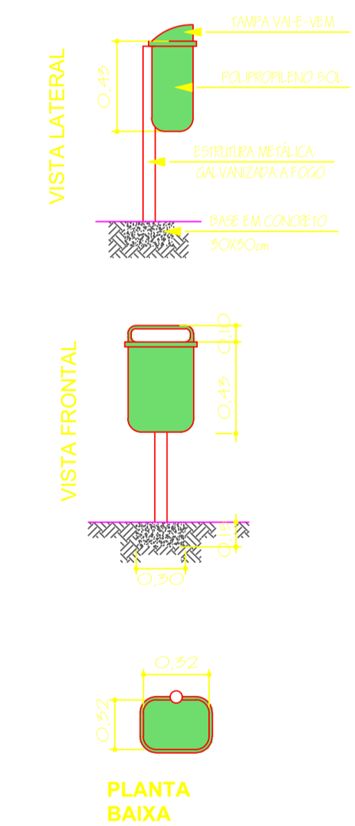
DETALHE LIXEIRA ESCALA: 1/25
