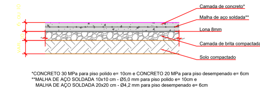
DETALHE GENÉRICO PISO CONCRETO ESCALA 1:25
