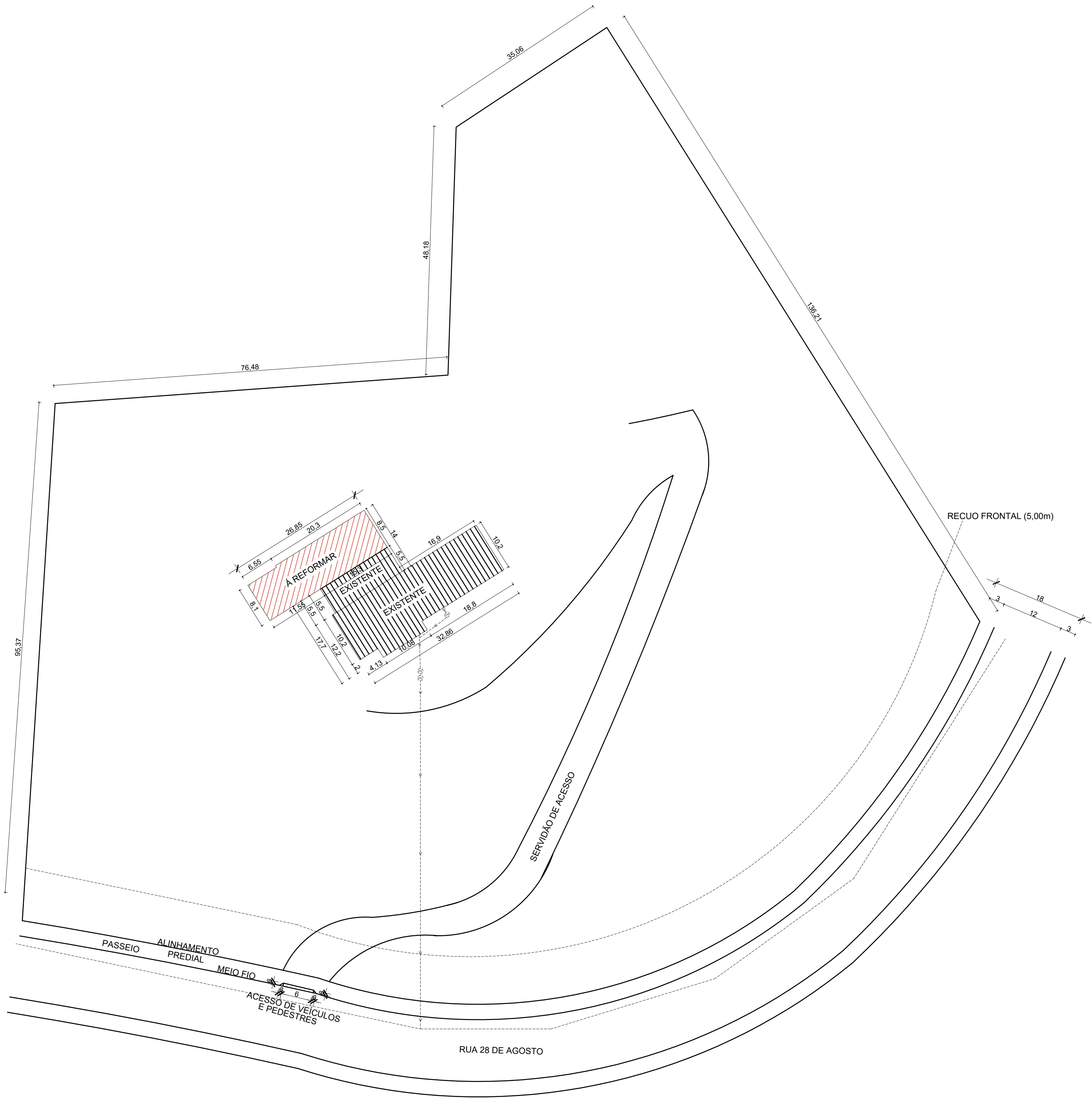
PLANTA DE LOCAÇÃO Esc.: 1/500
