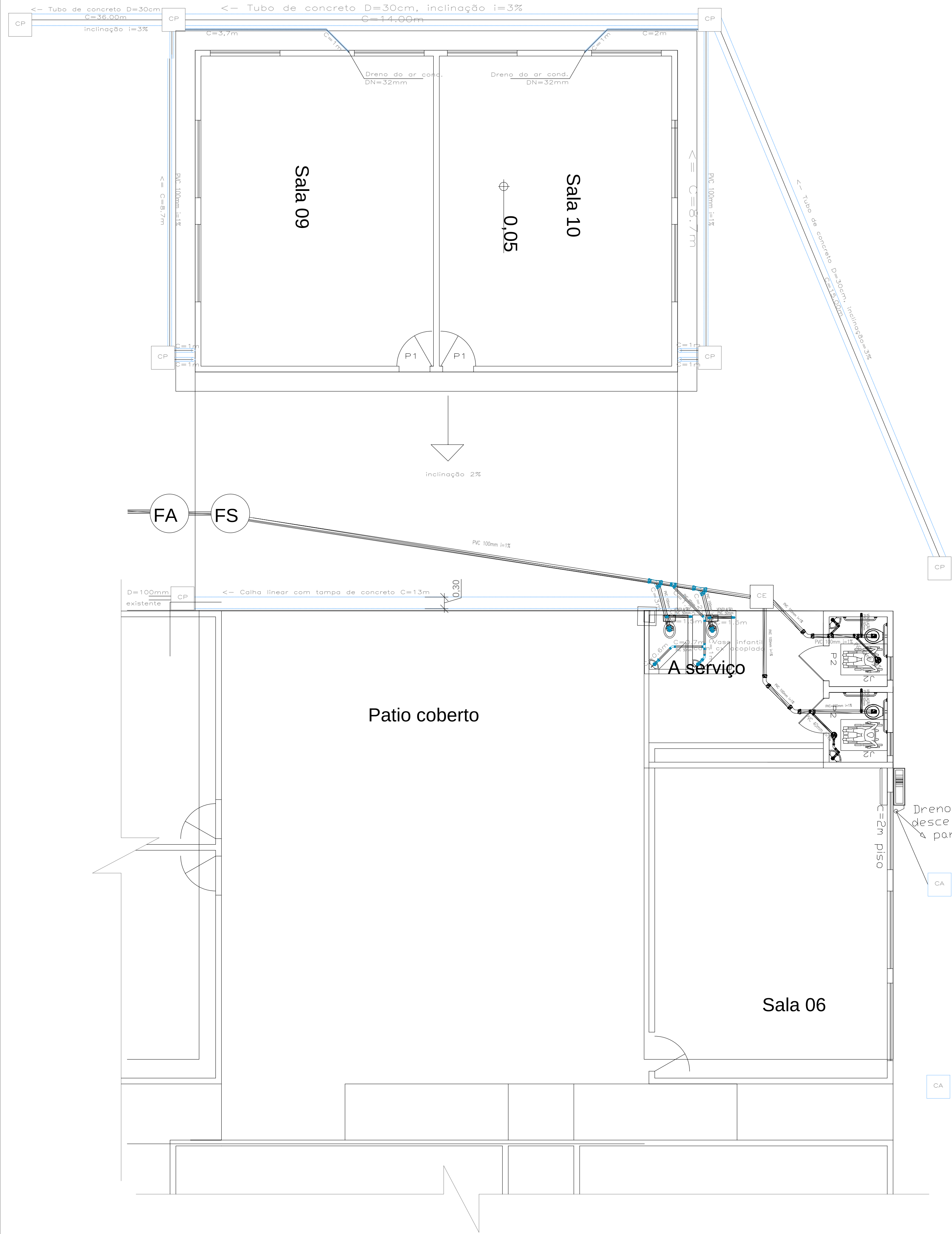
1 PLANTA BAIXA (ESGOTO E DRENAGEM PLUVIAL) ESC. 1/100
