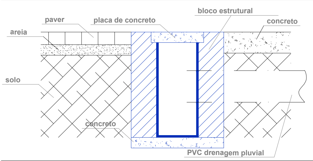
Detalhe 2 - CORTE DAS CALHAS DE PISO
