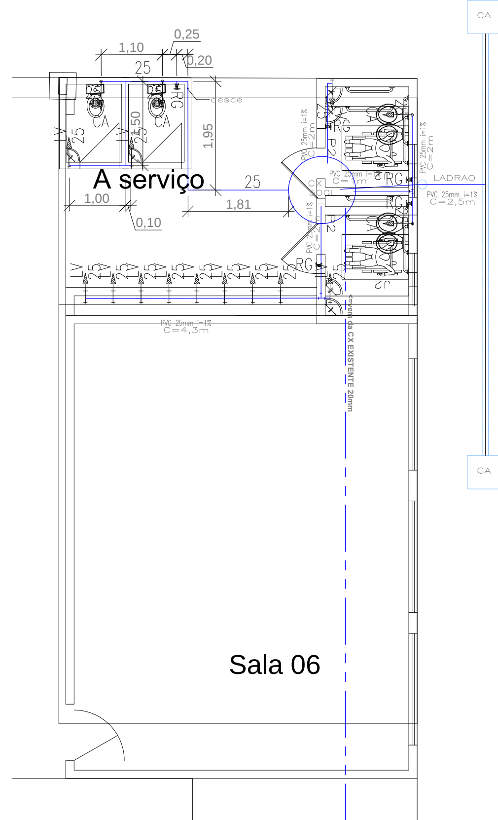
1 PLANTA BAIXA (AGUA FRIA) ESC. 1/100
