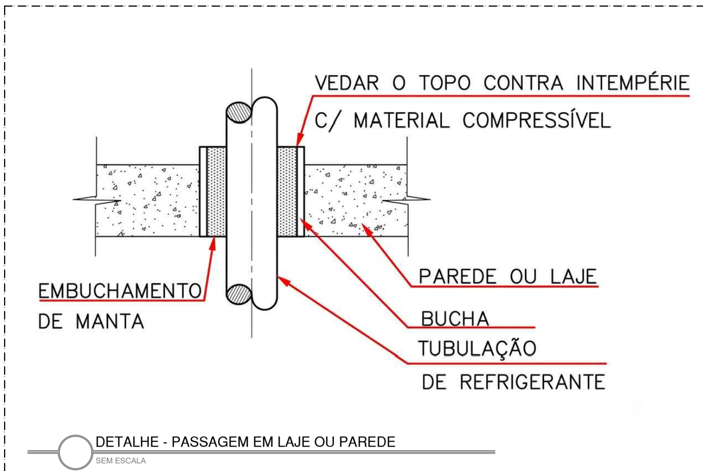
DETALHE - TUBULAÇÃO DE REFRIGERANTE
