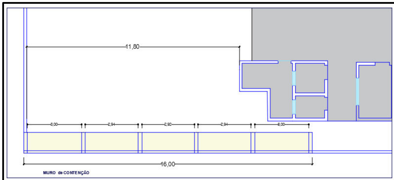
Planta do muro.
