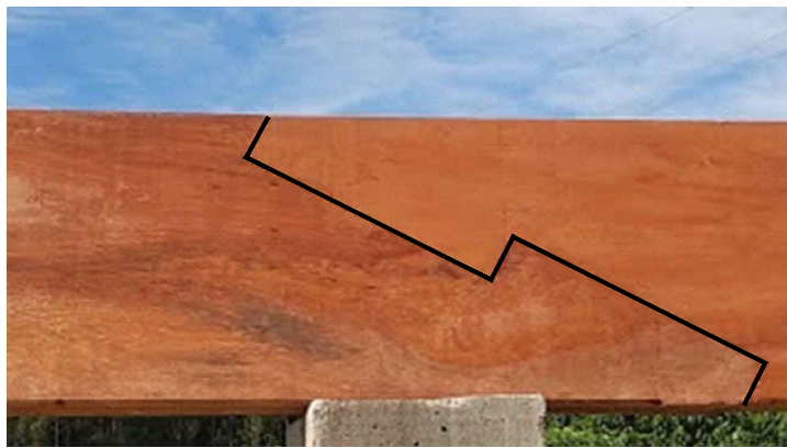
EMENDA DAS TERÇAS
