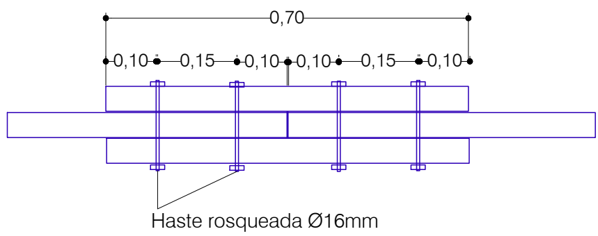
EMENDAS DOS CAIBROS
