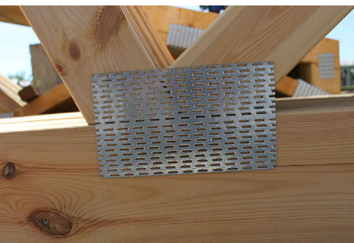
Conexões entre as peças: Anti-racha
