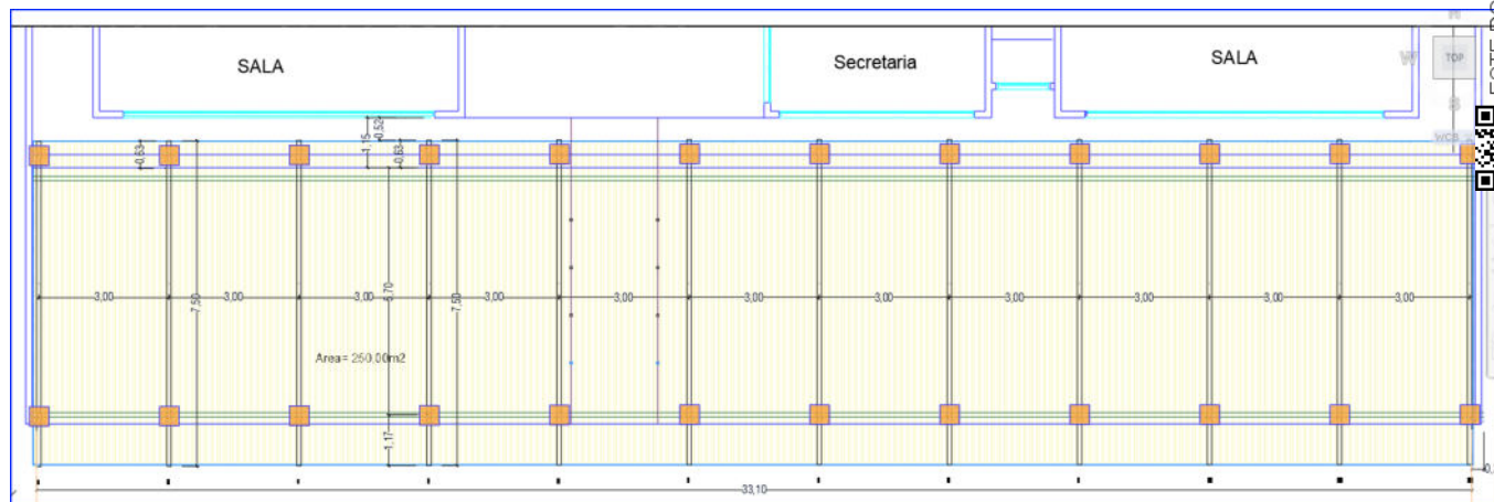
Planta da cobertura
