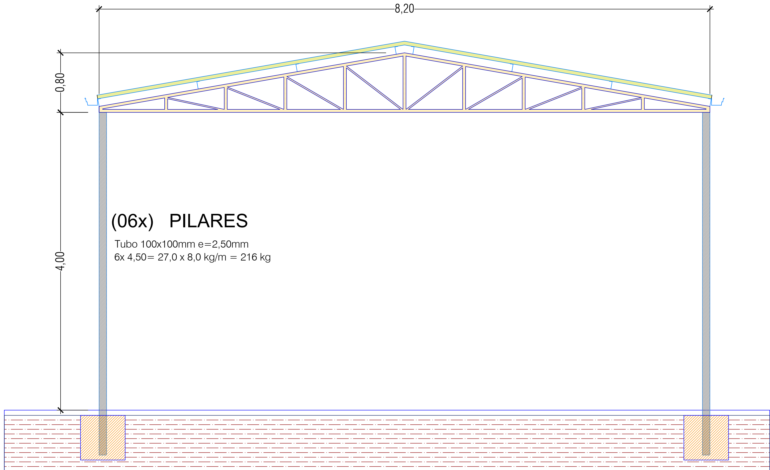
CORTE TRANSVERSAL
