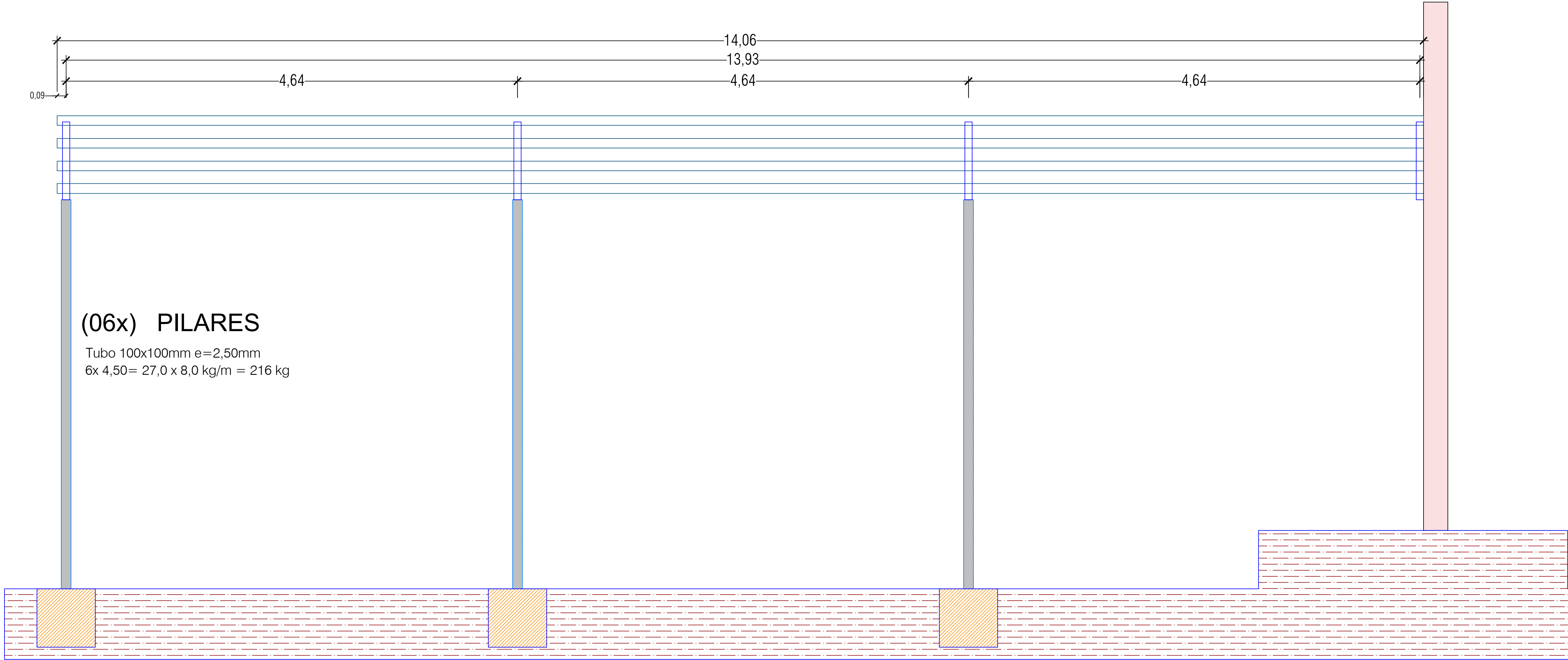
CORTE LONGITUDINAL
