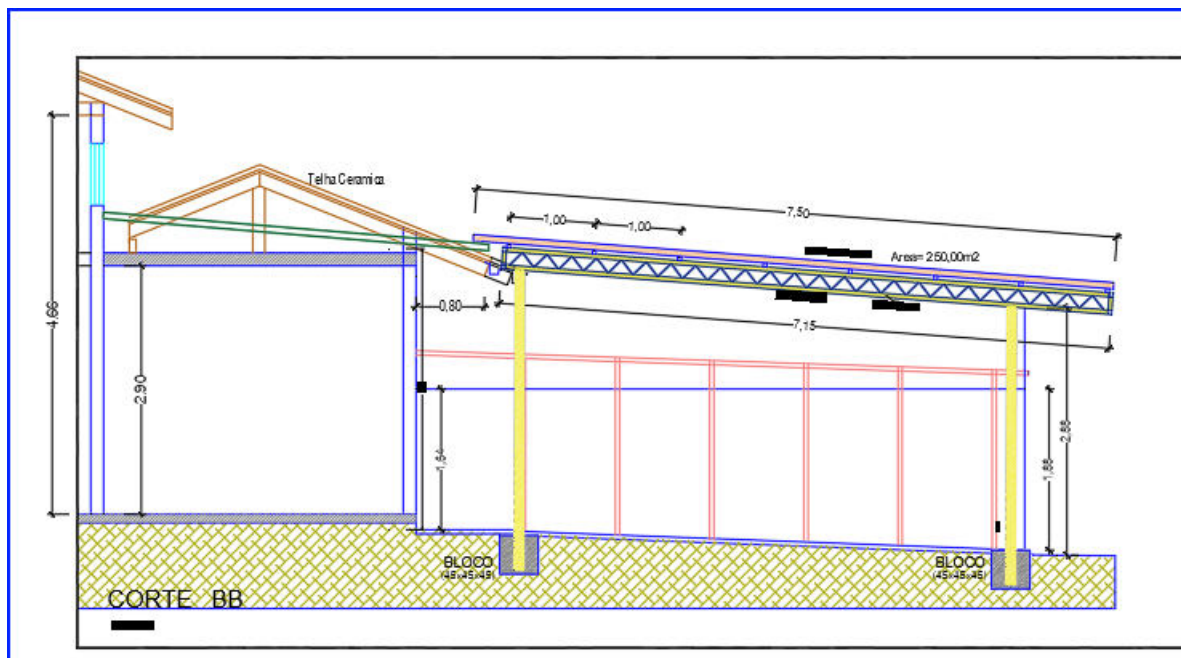
Seção transversal da estrutura.
