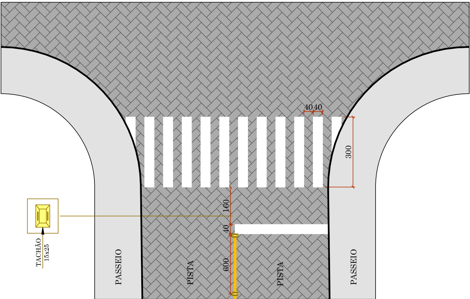
FAIXA PARA PEDESTRE – TIPO 01 PARA VIAS EM PAVIMENTO DE PAVER
