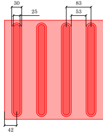
SINALIZAÇÃO TÁTIL DIRECIONAL
