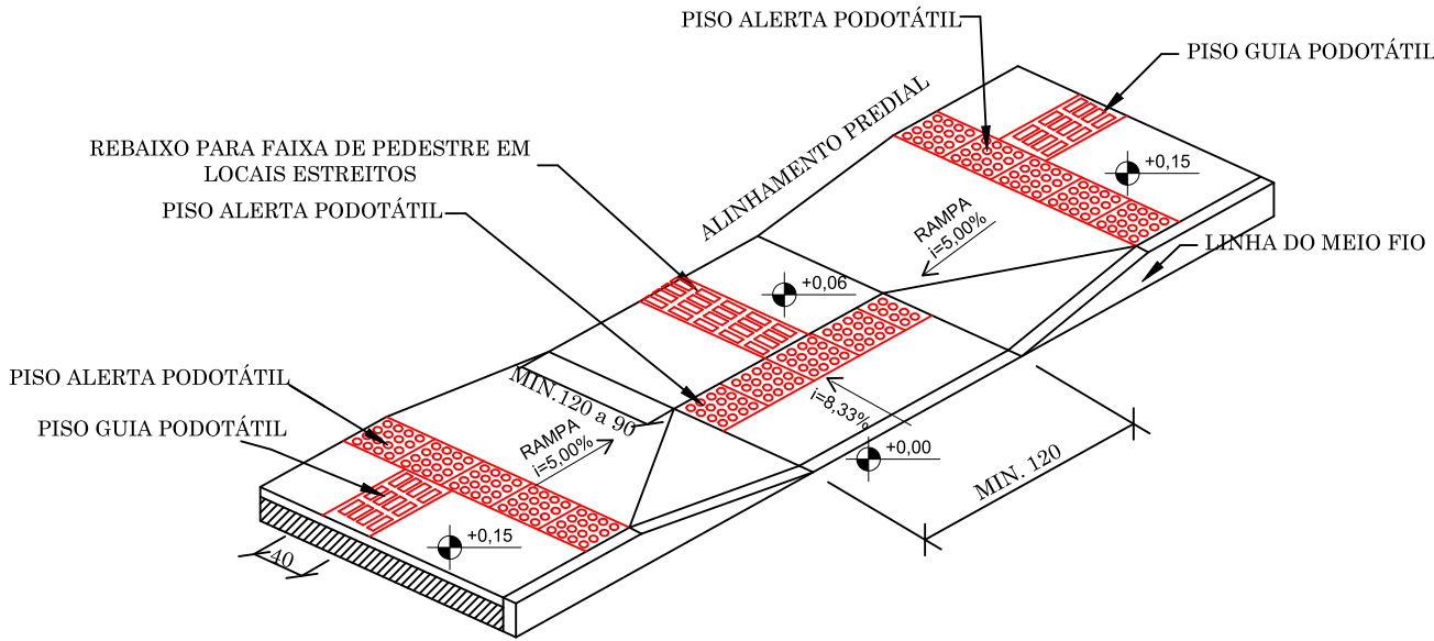
REBAIXO PARA TRAVESSIA DE PEDESTRES CALÇADA ESTREITA
