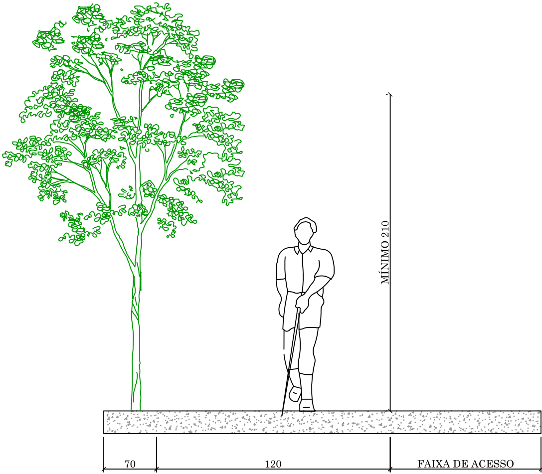
DETALHE FAIXA LIVRE
