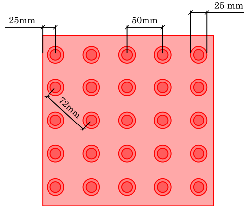
SINALIZAÇÃO TÁTIL DE ALERTA
