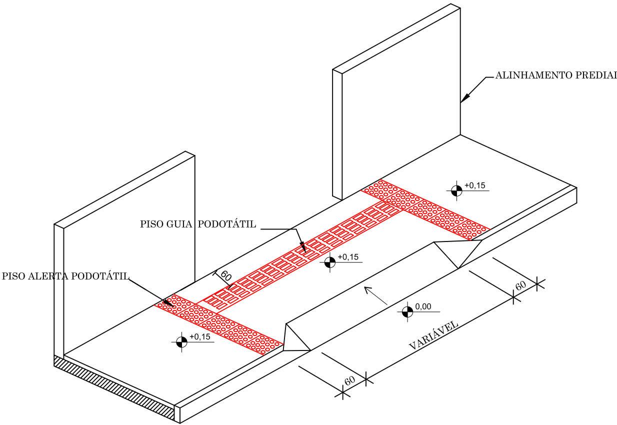
REBAIXO PARA ACESSO DE VEÍCULOS PARA LARGURA ≥ 140 cm
