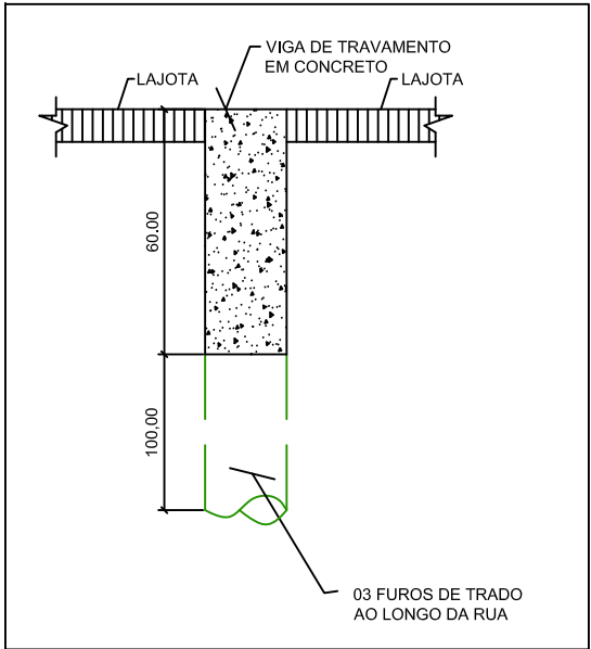
FUROS DE TRADO:
