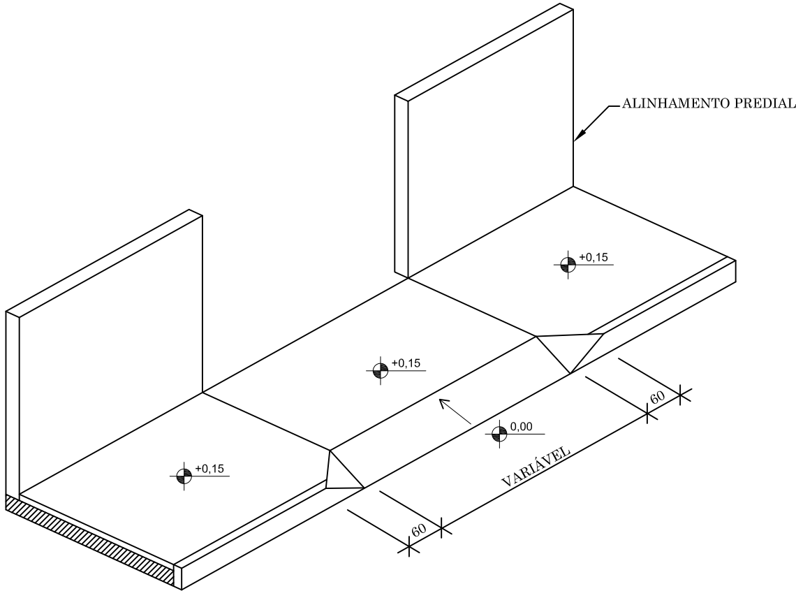
REBAIXO PARA ACESSO DE VEÍCULOS
