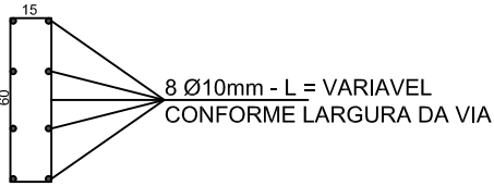
CORTE AA
