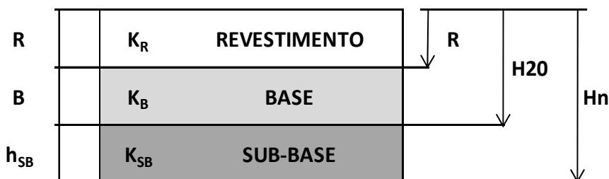
Figura 6 – Representação das Camadas estruturais do pavimento.
