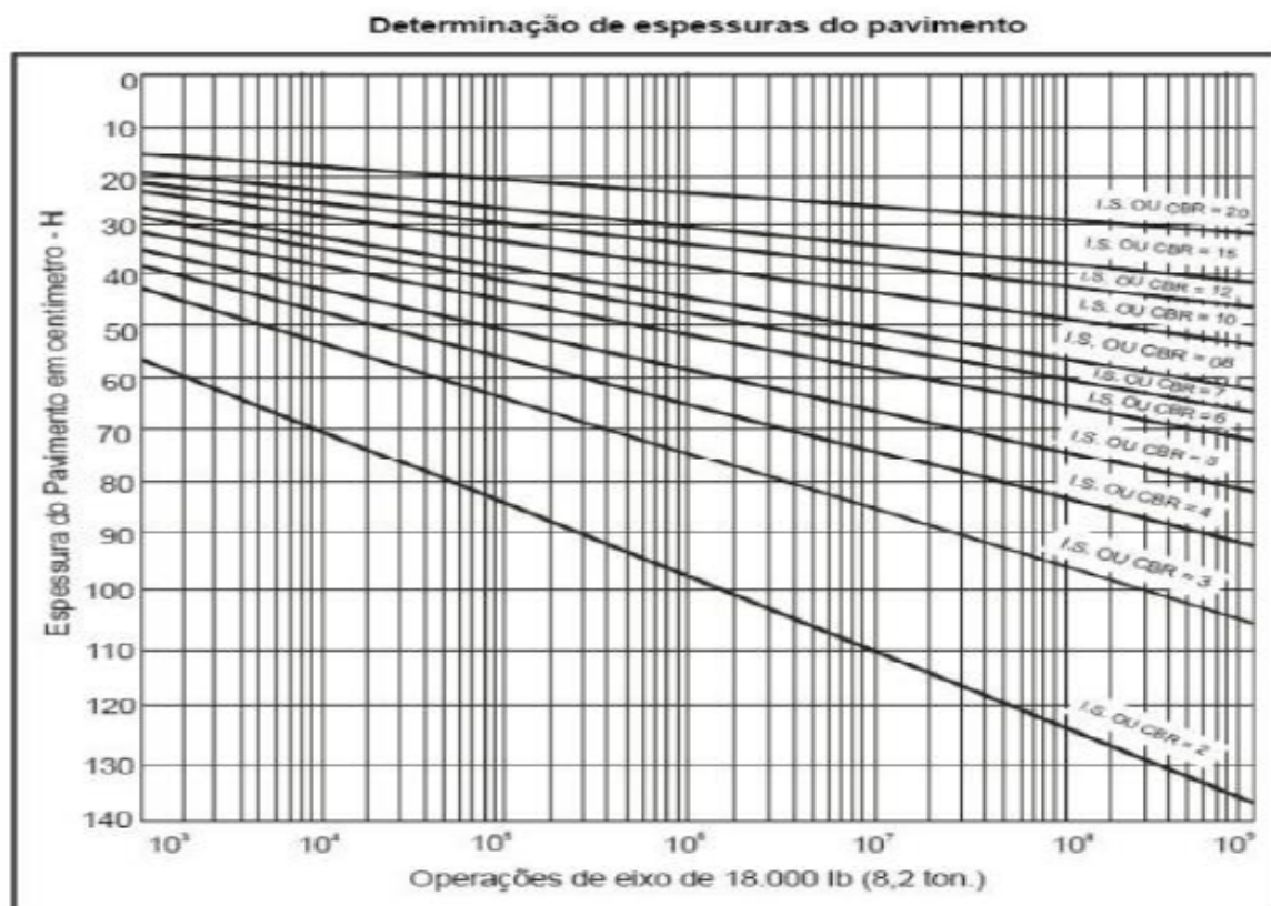
Figura 5 – Ábaco para determinação das espessuras do pavimento
