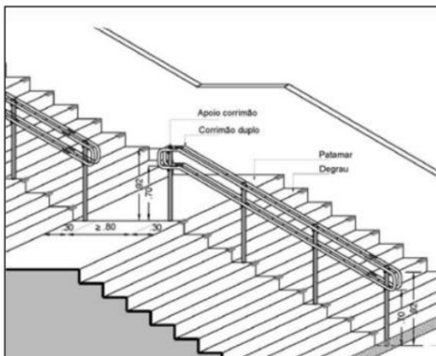
Figura 3: Corrimão duplo - Escadas arquibancadas.
