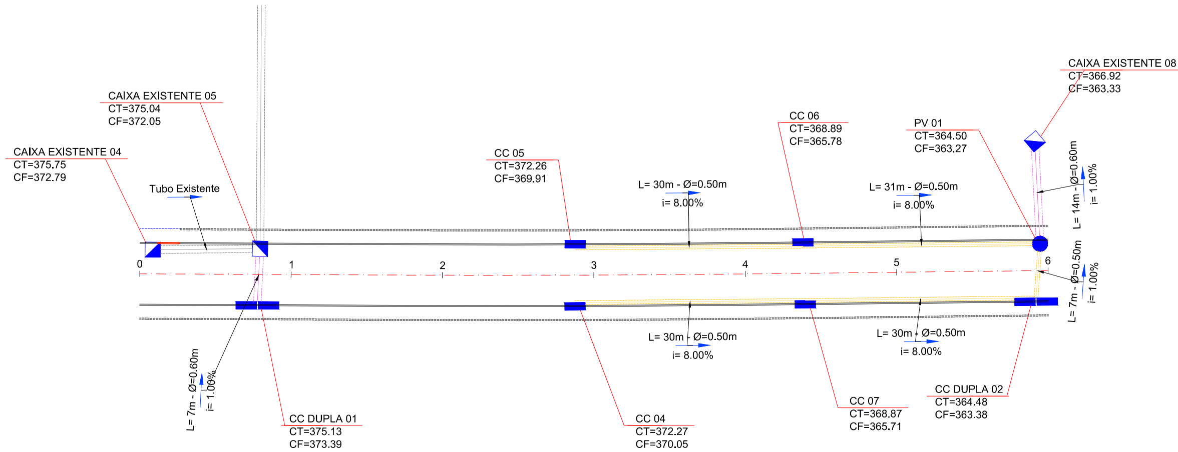
Planta Baixa - Rua Luigi Chirolli Est: 0+0.00 à 6+0.000 Esc: 1/500
