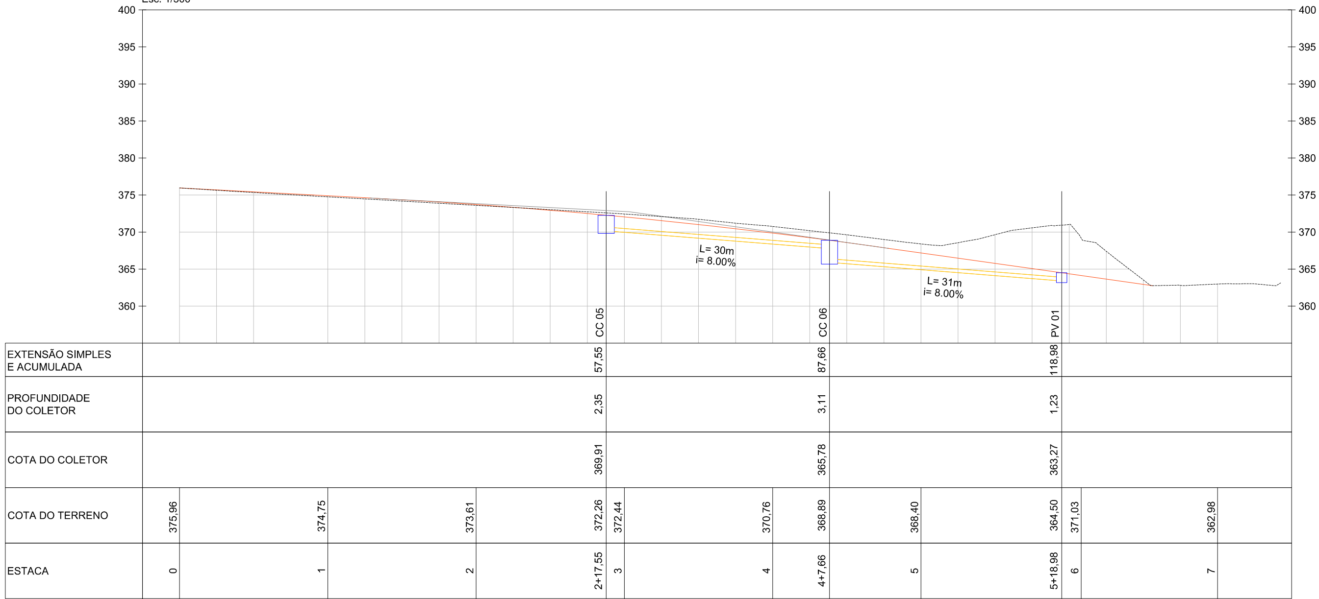
Perfil Drenagem - Rua Luigi Chirolli (Lado Direito) Est: 0+0.00 à 7+10.00 Esc: 1/500
