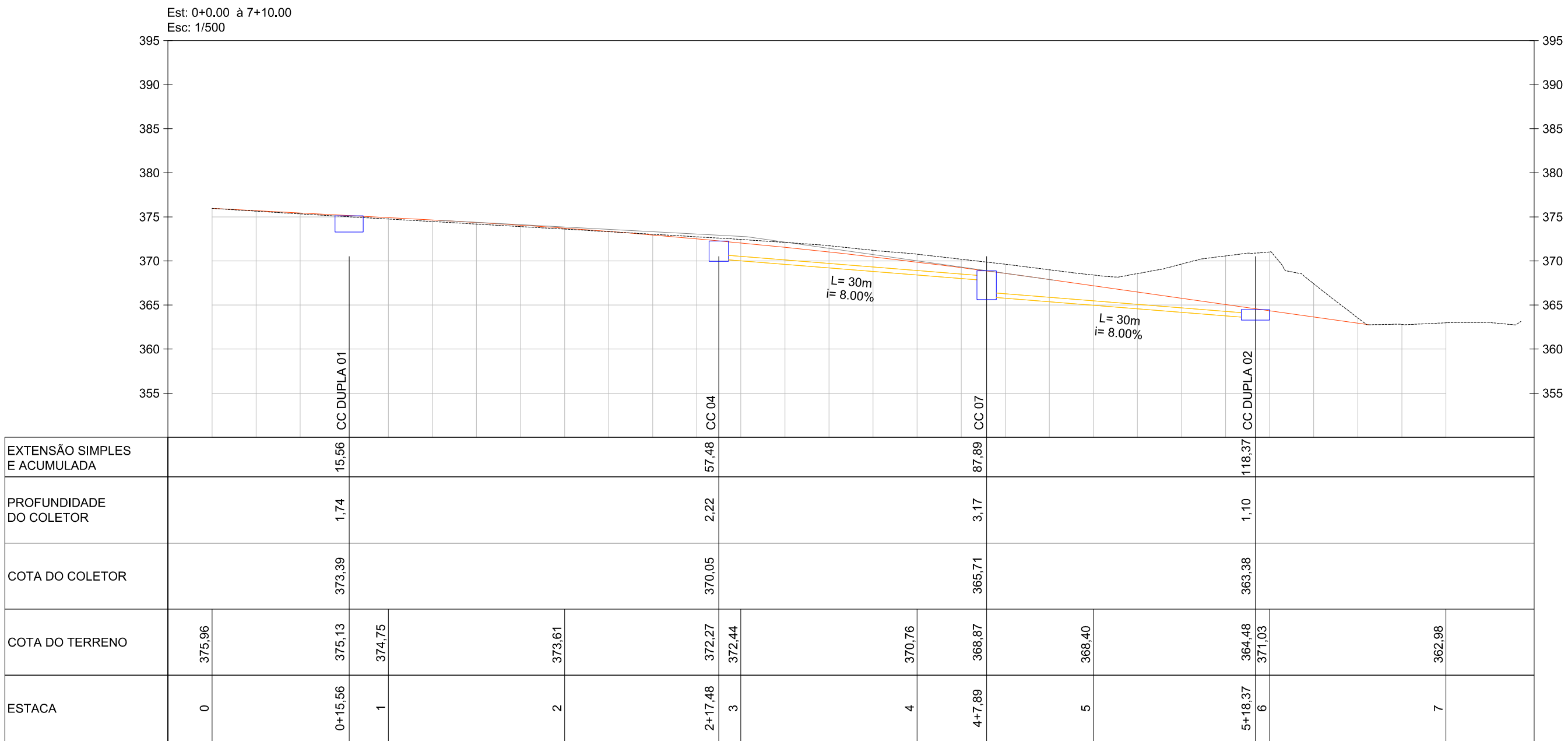
Perfil Drenagem - Rua Luigi Chirolli (Lado Direito) Est: 0+0.00 à 7+10.00 Esc: 1/500
