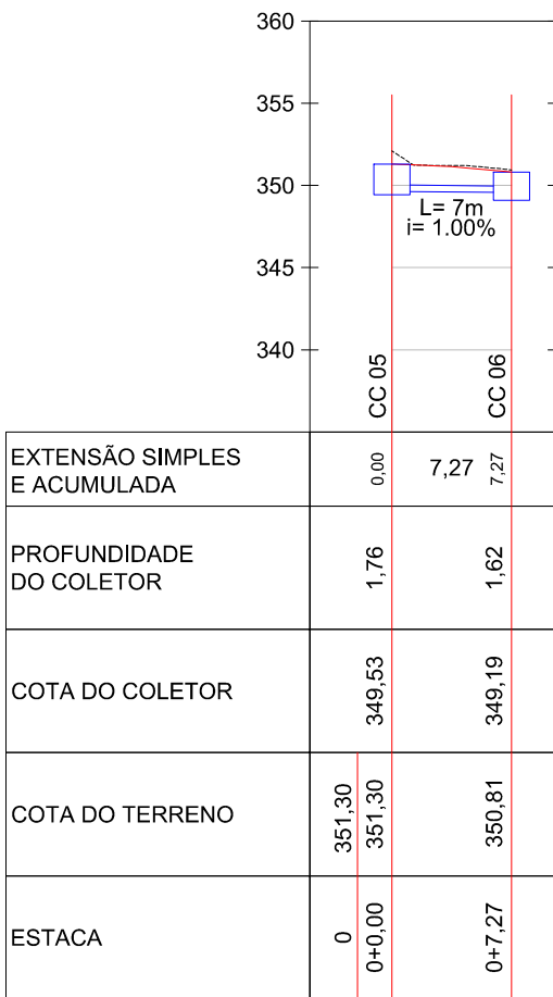
Travessia 03 0+0,00 à 0+10,00 Esc: 1/500
