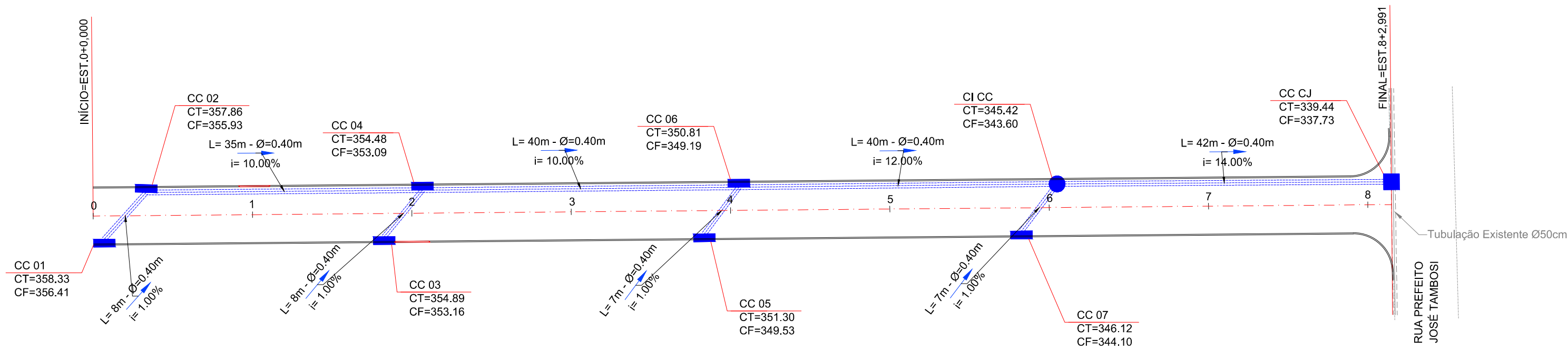
Planta Baixa - Rua Irmã Maria Avosani Est. 0 + 0,00 à 8 + 2,991 Esc: 1/500
