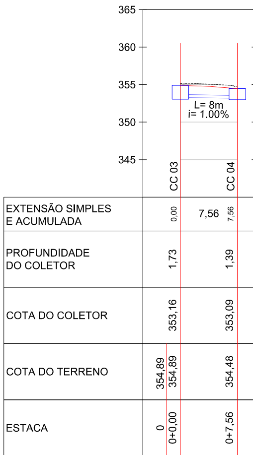
Travessia 02 0+0,00 à 0+10,00 Esc: 1/500
