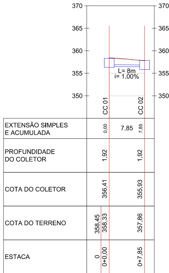
Travessia 01 0+0,00 à 0+10,00 Esc: 1/500
