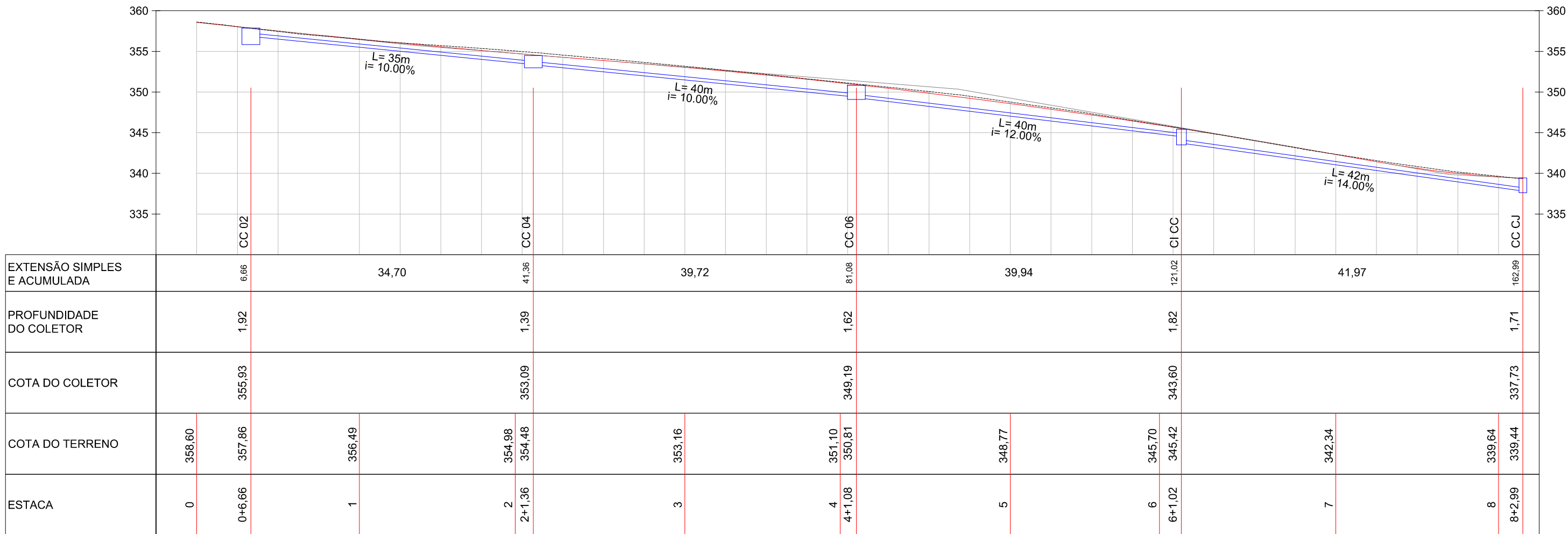
Perfil Drenagem - Rua Irmã Maria Avosani 0+0,00 à 8+5,00 Esc: 1/500
