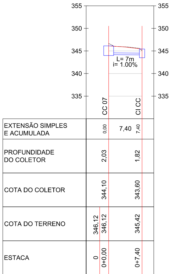
Travessia 04 0+0,00 à 0+10,00 Esc: 1/500
