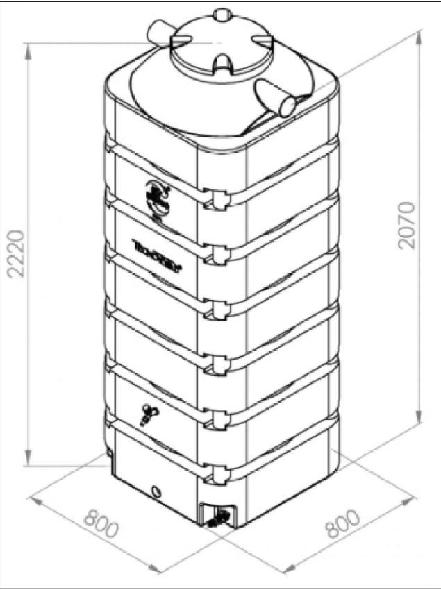
DETALHE CISTERNA
