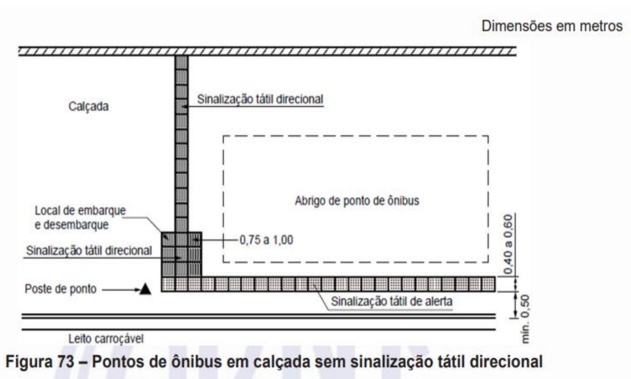
Figura 73 da ABNT NBR 16537/2024 referente à instalação de piso tátil em pontos de ônibus
