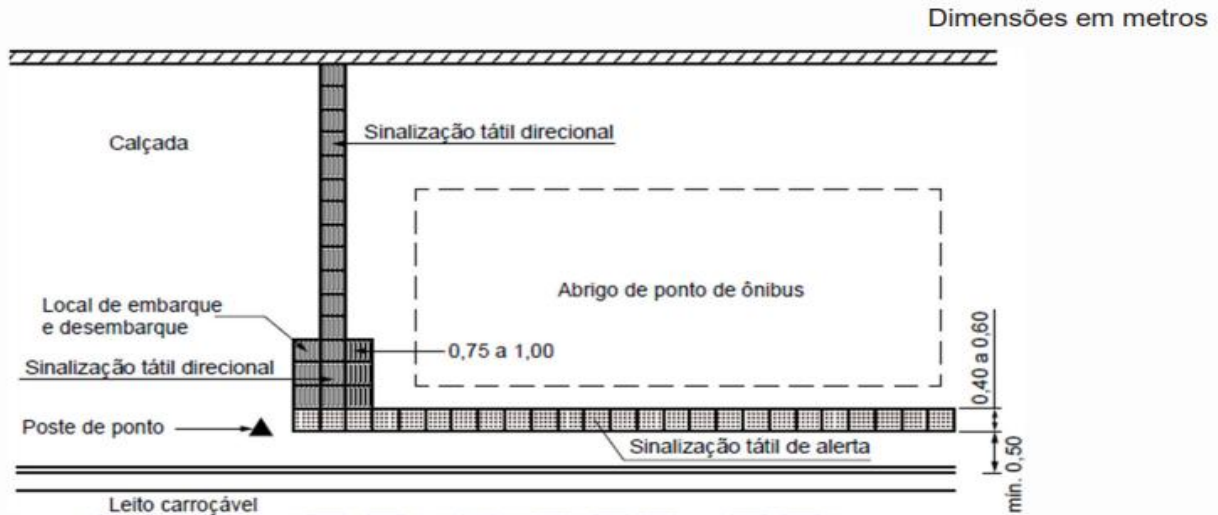
Figura 73 – Pontos de ônibus em calçada sem sinalização tátil direcional
