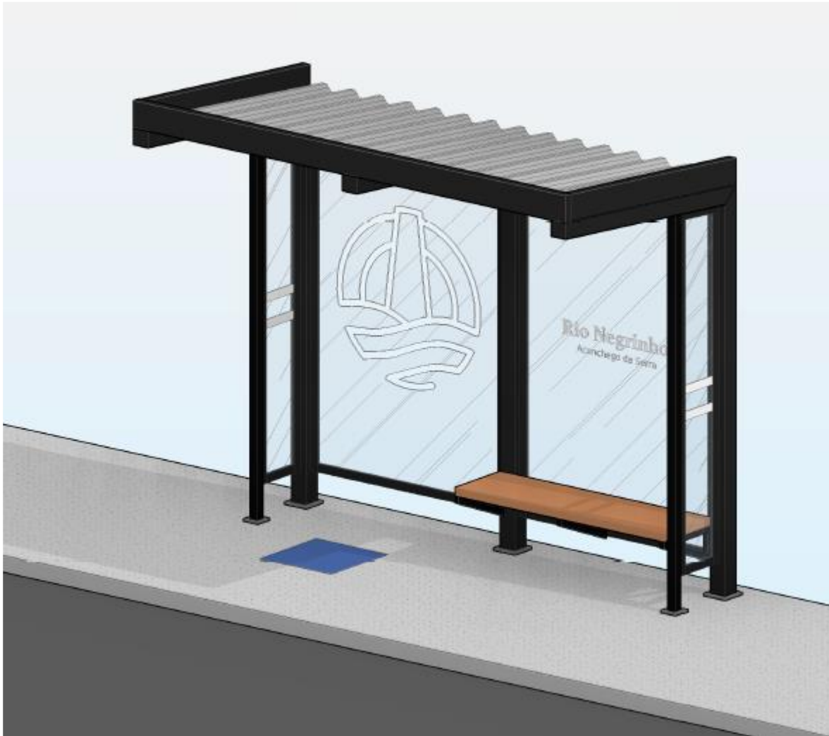
Figura 1 – Modelo 01 – Lateral 0,50 m
