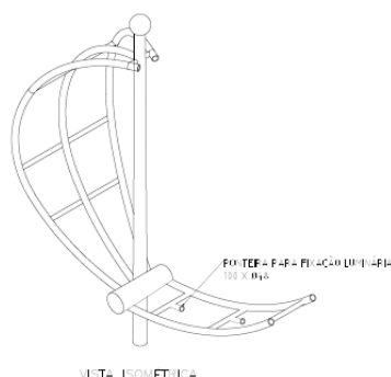
Novo modelo de suporte em Vela
