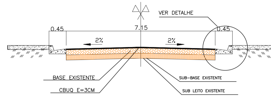
TRAV. JARBAS PASSARINHO TRECHO JB 2 SEÇÃO TRANSVERSAL S/ ESCALA
