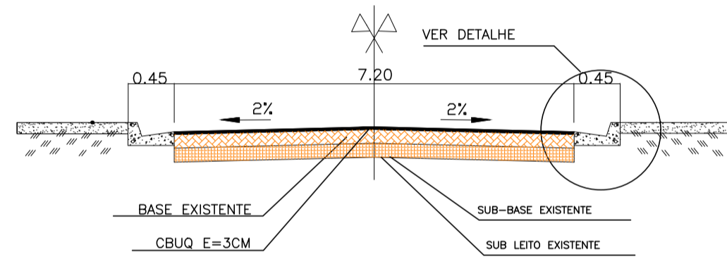
TRAV. JARBAS PASSARINHO TRECHO JB 1 SEÇÃO TRANSVERSAL S/ ESCALA
