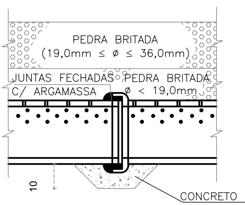
JUNTAS DOS TUBOS DETALHE ESCALA 1:20
