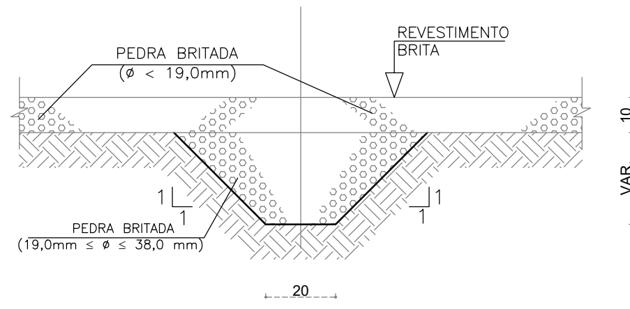
VALETA PARA CAPTAÇÃO DE ÁGUAS ESCALA 1:20
