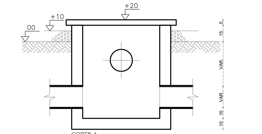
CORTE A SEM ESCALA
