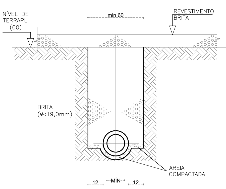
DETALHE VALA TUBO POROSO ESCALA: 1:20
