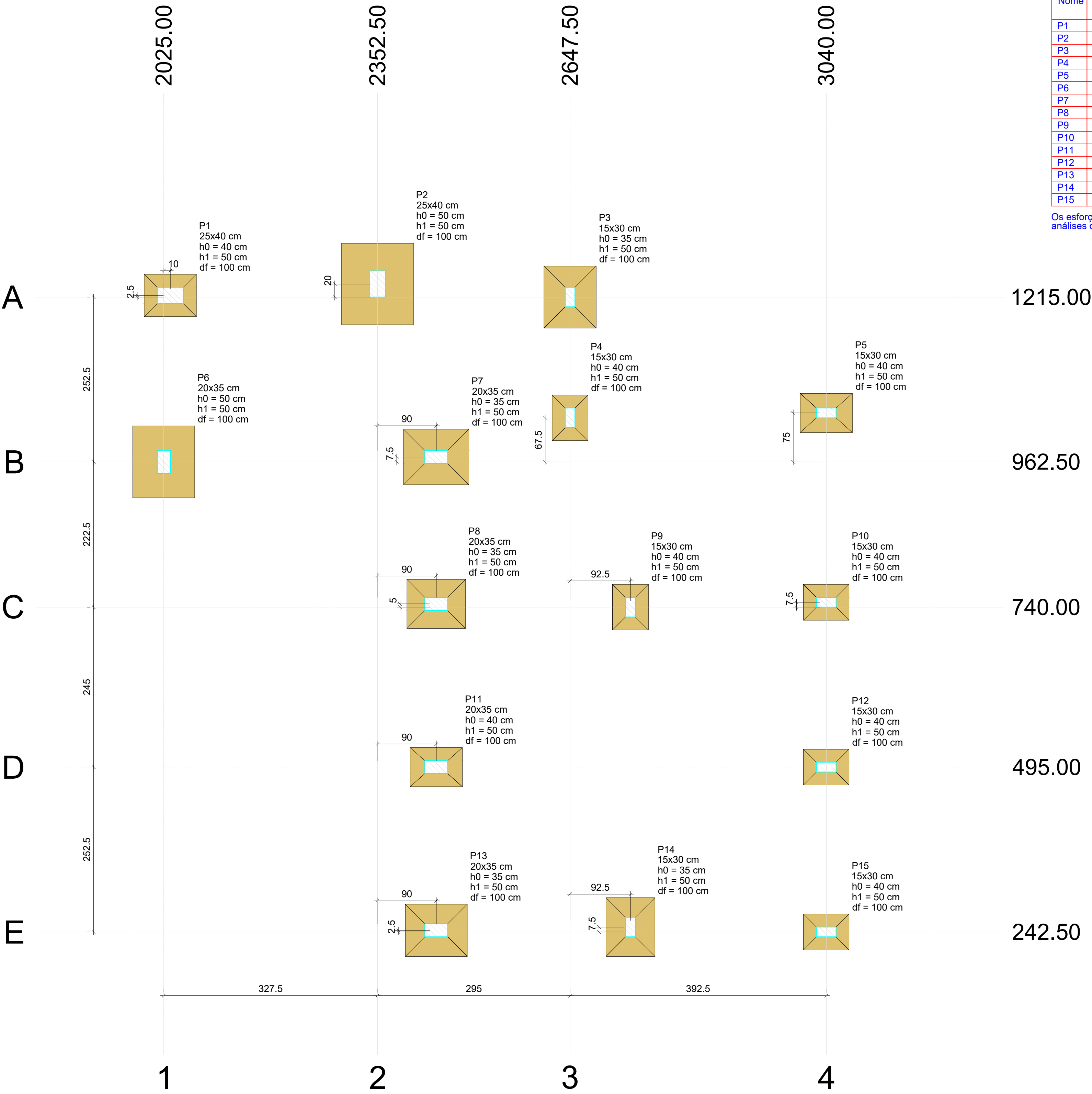
PLANTA DE LOCAÇÃO Escala 1:75
