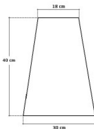
Figura 2: Perfil do marco piramidal padrão IBGE (fonte: Padronização de Marcos Geodésicos - IBGE)
