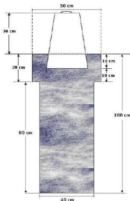
Figura 4: Esquema de estabelecimento de marco padrão IBGE (fonte: Padronização de Marcos Geodésicos - IBGE)
