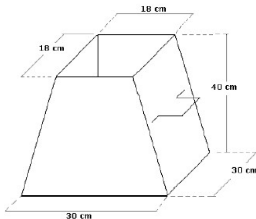
Figura 3: Forma com os padrões utilizados para o marco piramidal padrão IBGE (fonte: Padronização de Marcos Geodésicos - IBGE)
