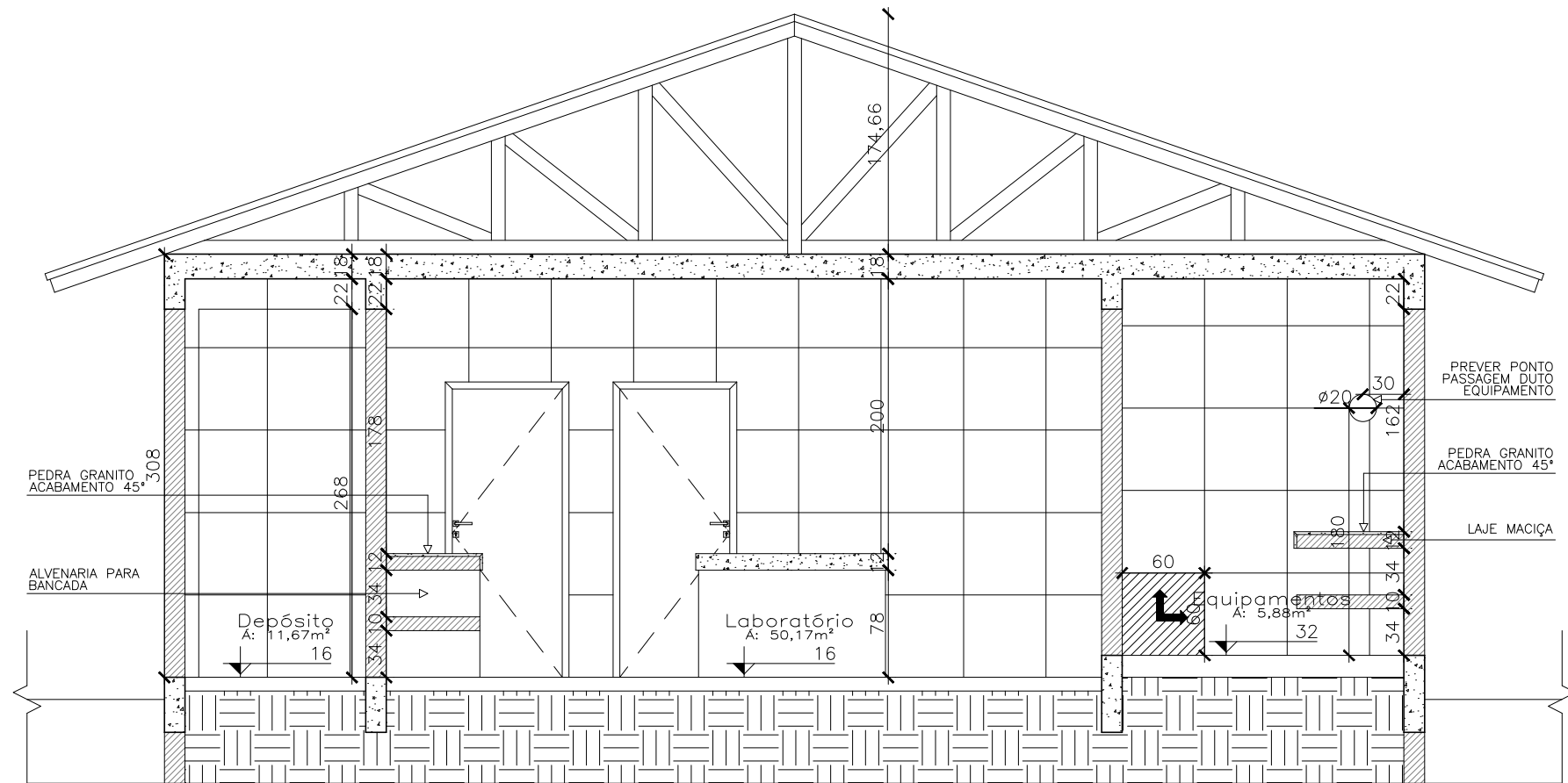
CORTE AA – DET. 05 ESC 1/50
