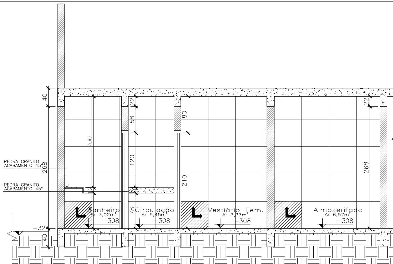
CORTE AA - DET. 04 ESC 1/50
