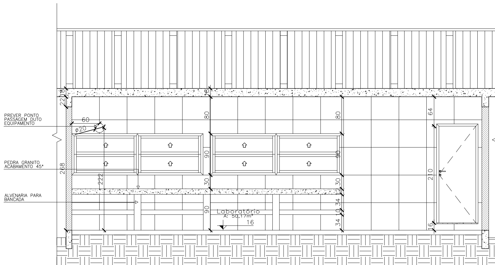
CORTE BB – DET. 05 ESC 1/50
