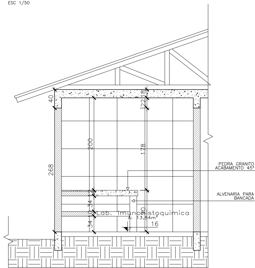
CORTE BB - DET. 07 ESC 1/50
