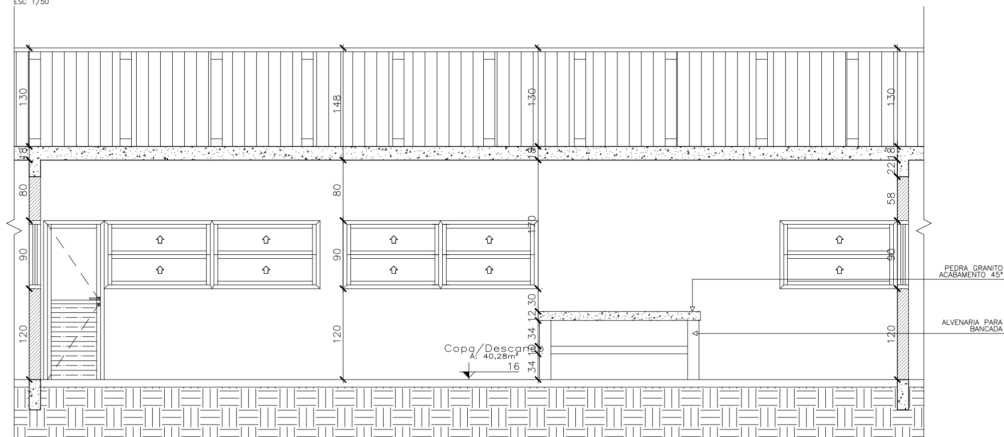
CORTE AA - DET. 08 ESC 1/50
