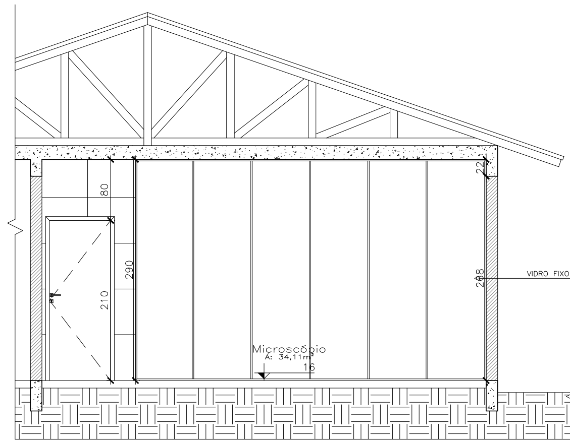
CORTE AA - DET. 06 ESC 1/50
