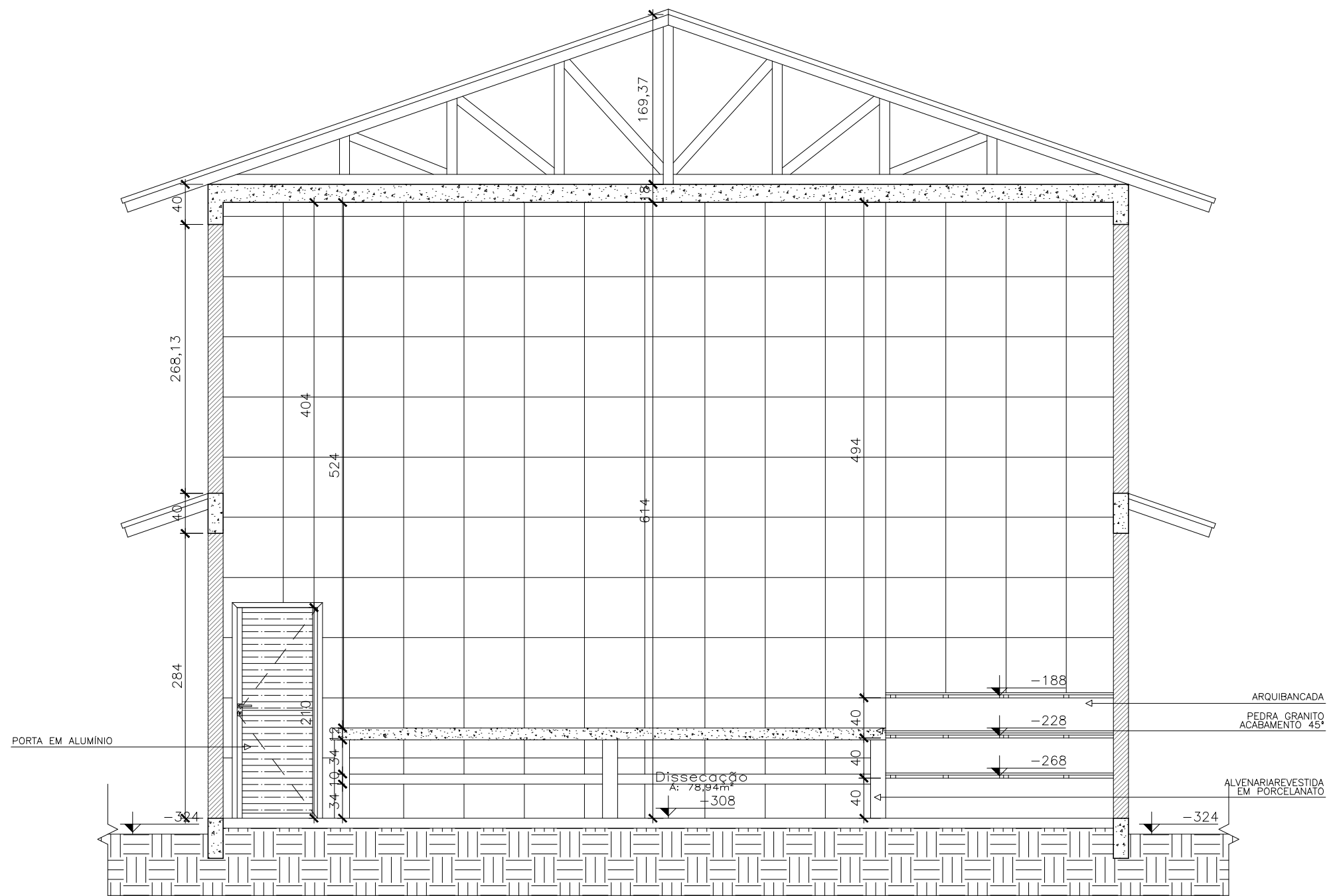
CORTE BB - DET. 03 ESC 1/50
