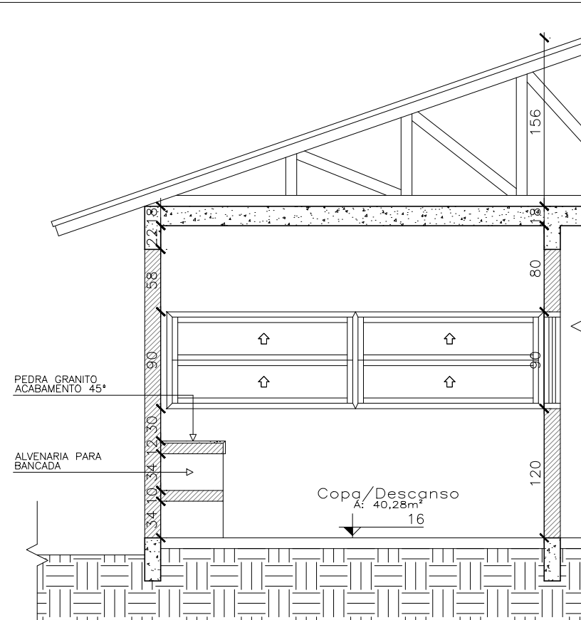
CORTE AA - DET. 08 ESC 1/50
