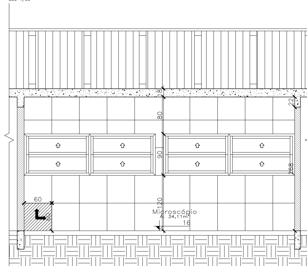
CORTE BB - DET. 06 ESC 1/50
