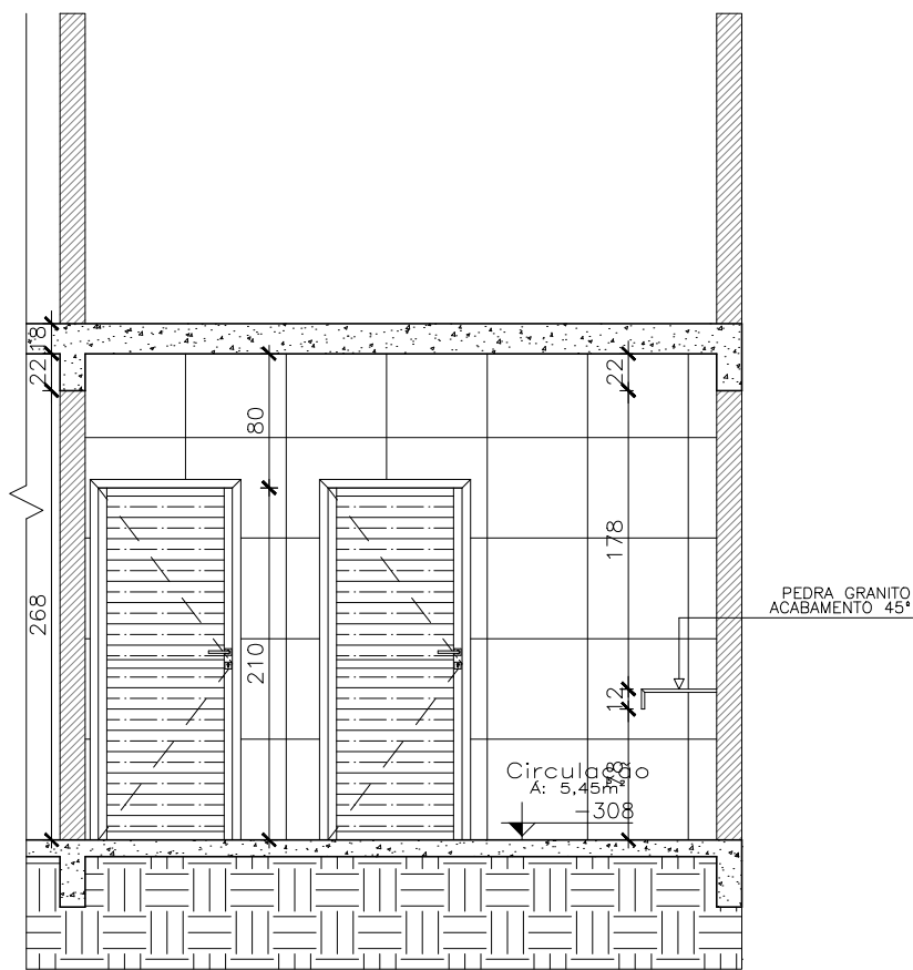
CORTE BB - DET. 04 ESC 1/50
