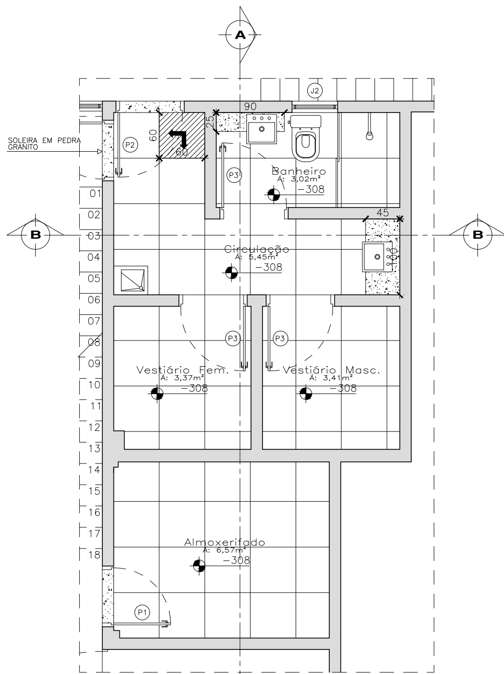
DETALHAMENTO 04 ESC 1/50
