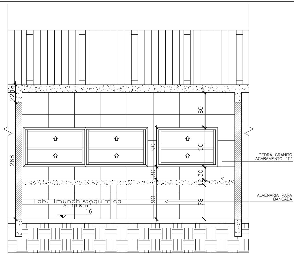
CORTE AA - DET. 07 ESC 1/50
