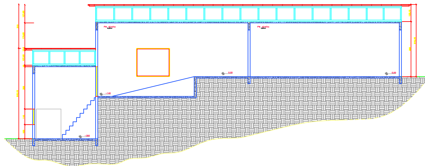
CORTE LONGITUDINAL AA' ESC 1/16
