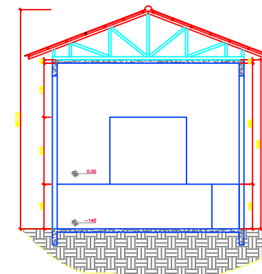
CORTE TRANSVERSAL BB' ESC 1/16
