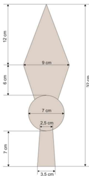
LANÇA (ACABAMENTO NIQUELADO)
