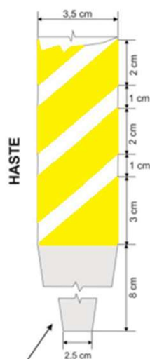
CONTO (parte inferior da haste) ACABAMENTO NIQUELADO
