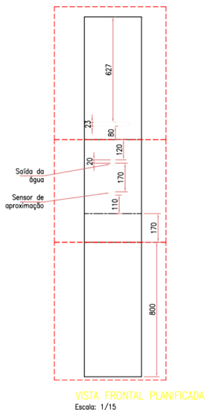
Imagem 02 – Dimensões orientativas do equipamento.
