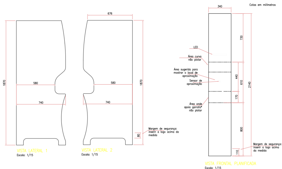
Imagem 01 – Dimensões orientativas do equipamento.
