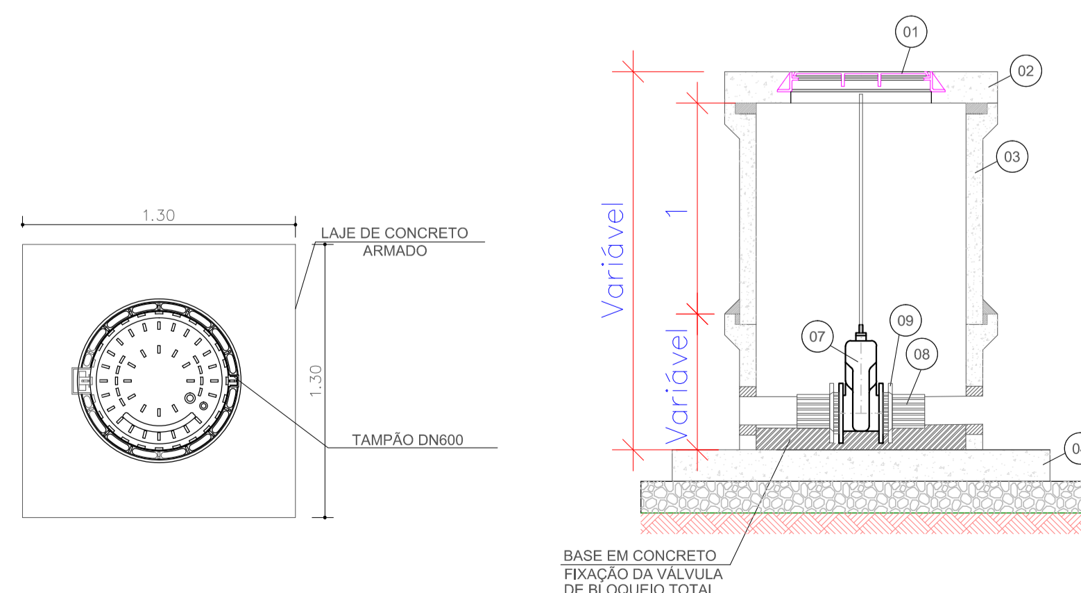
DETALHES DOS PVS ESCALA 1:25
