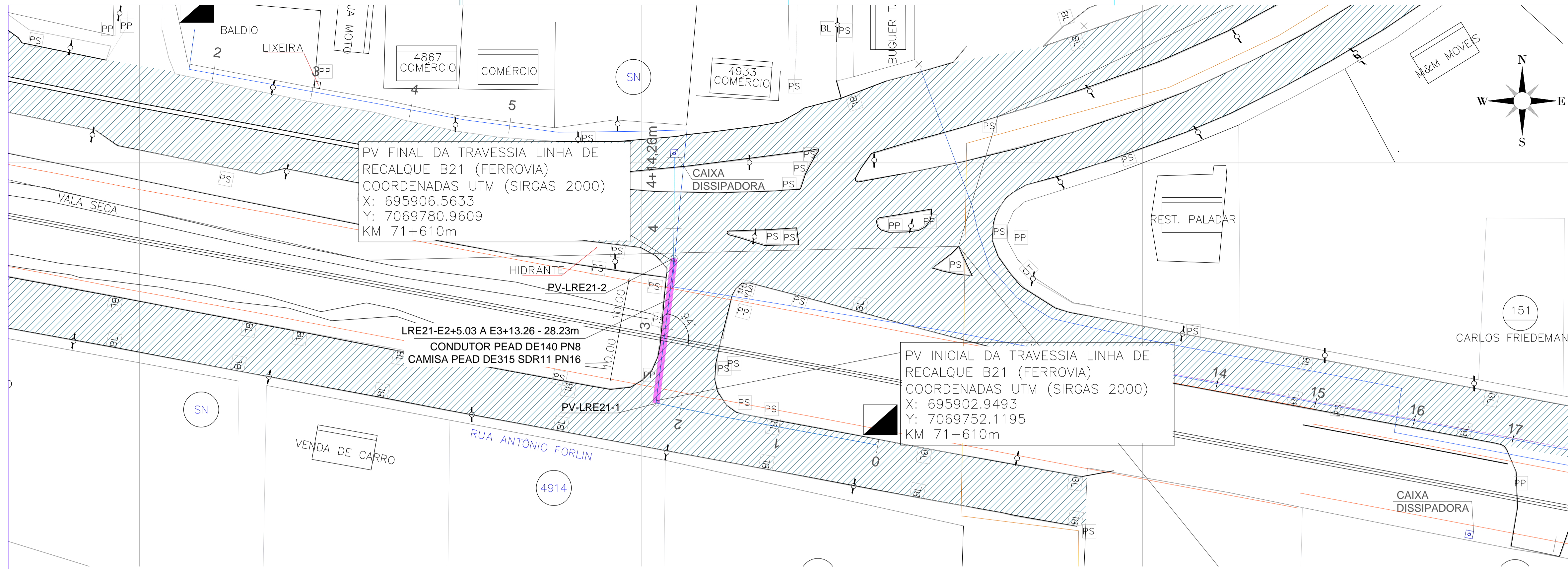
PLANTA BAIXA: TRAVESSIA B21 ESCALA 1:500
