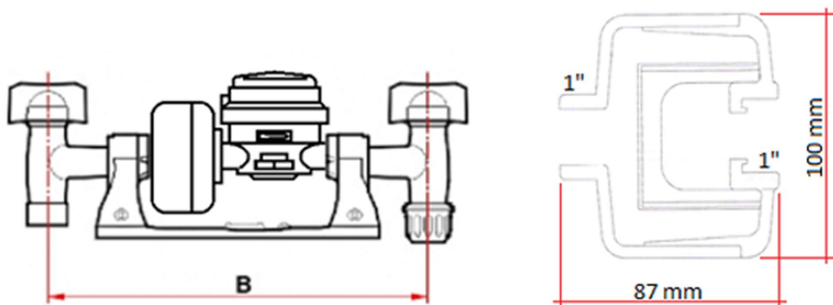
Figura 04: Corte lateral
