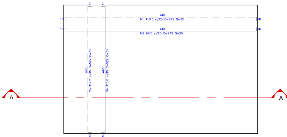
PLANTA BAIXA - ARMADURAS
