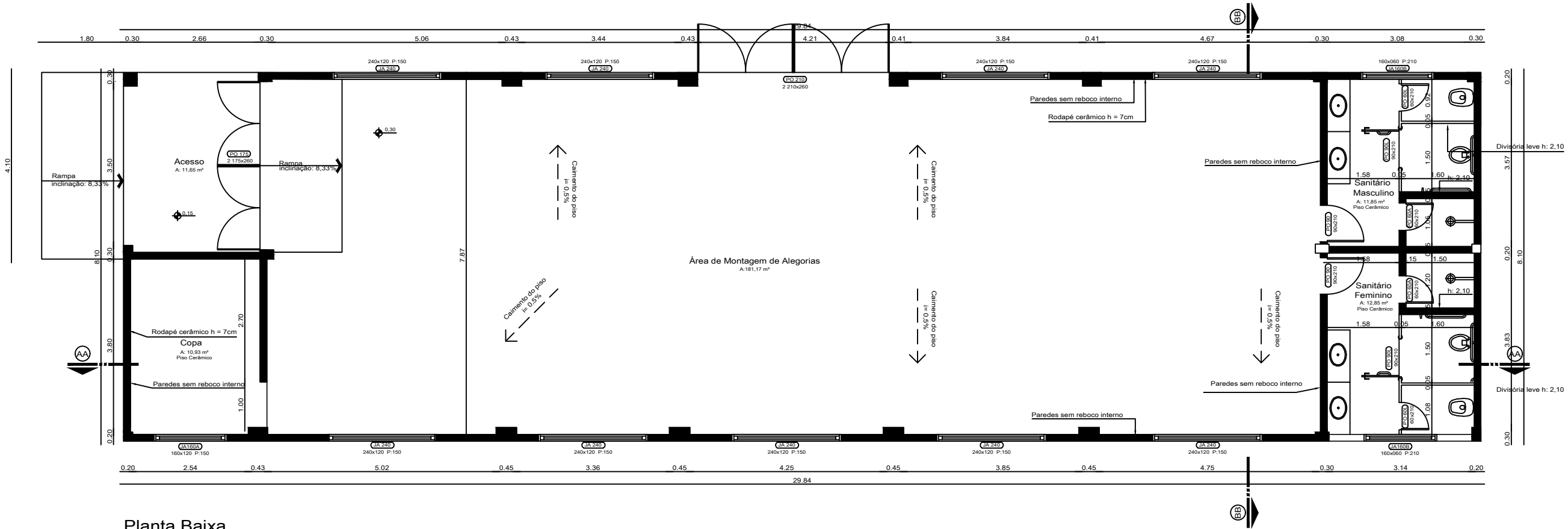
Planta Baixa
