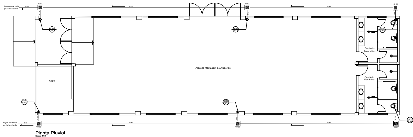
Planta Pluvial Escala 1:50
