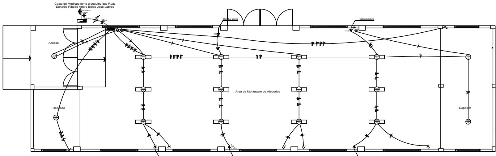
Planta Baixa Elétrico (superior) Escala 1/150
