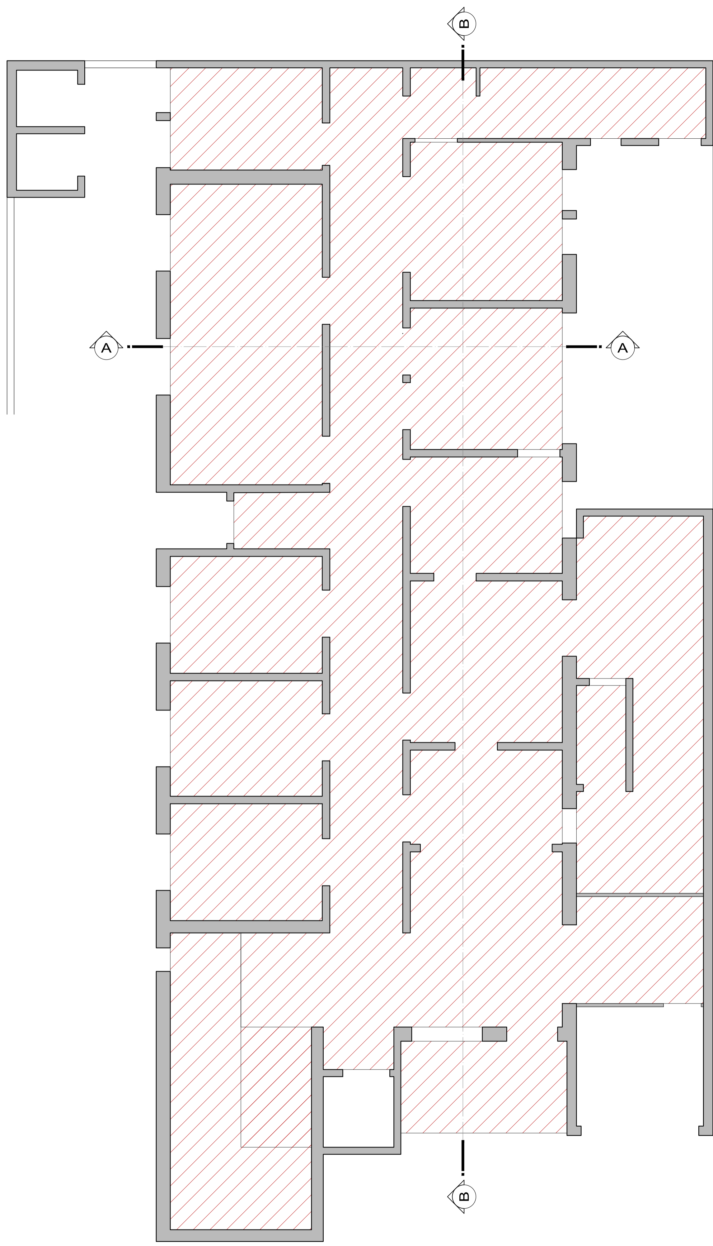
PAVTO. INFERIOR REFORMA PISO ESCALA 1/50 ÁREA DE PISO A DEMOLIR: 200,00m 2 (andar) + 17,68m 2 (escada) ÁREA DE PISO A INSTALAR: 220,00m 2 (andar) + 19,45m 2 (escada) | Considerando 10% de quebra
