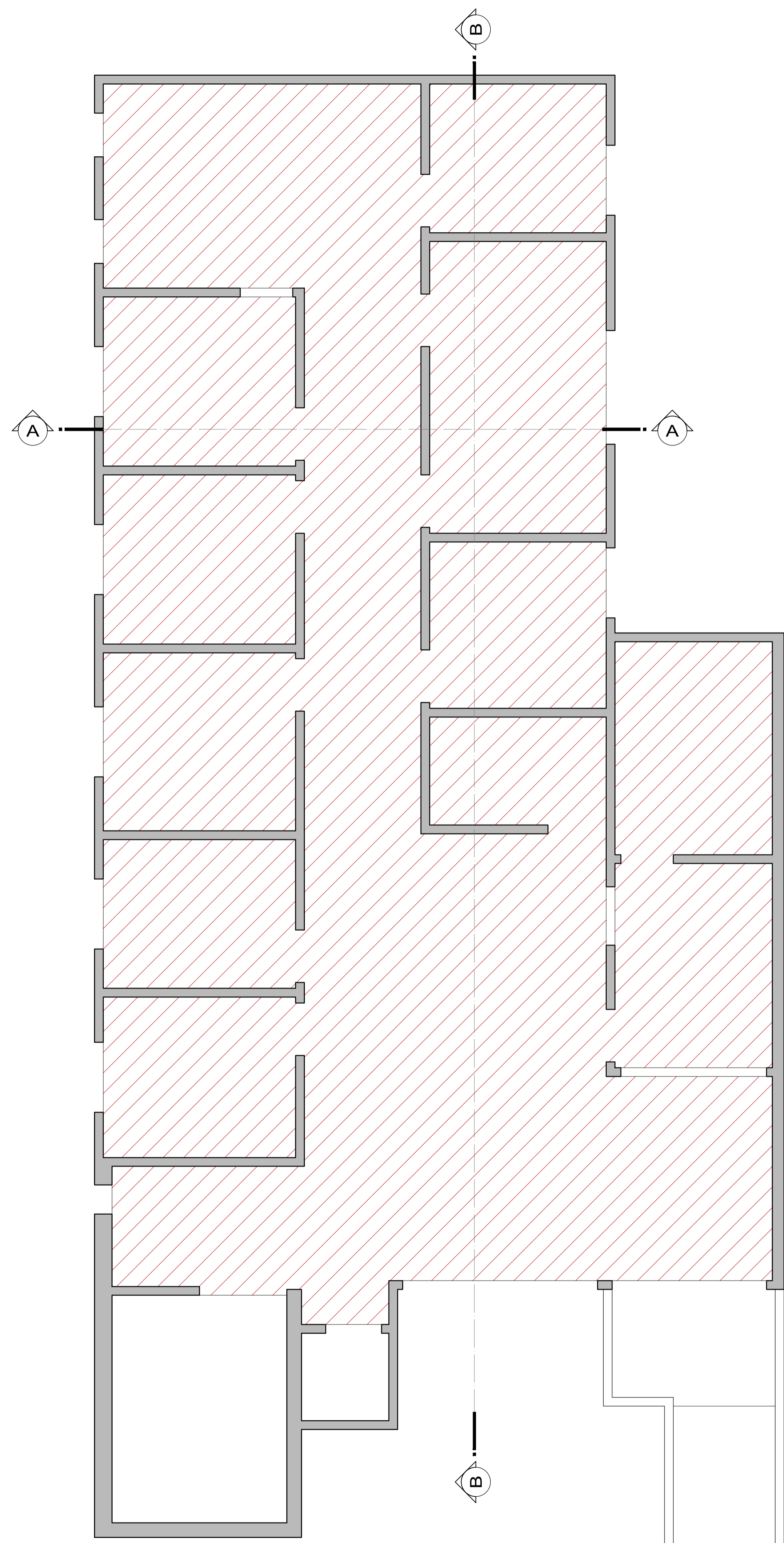
PAVTO. SUPERIOR REFORMA PISO ESCALA 1/50 ÁREA DE PISO A DEMOLIR: 200,00m 2 ÁREA DE PISO A INSTALAR: 220,00m 2 (considerando 10% de quebra)
