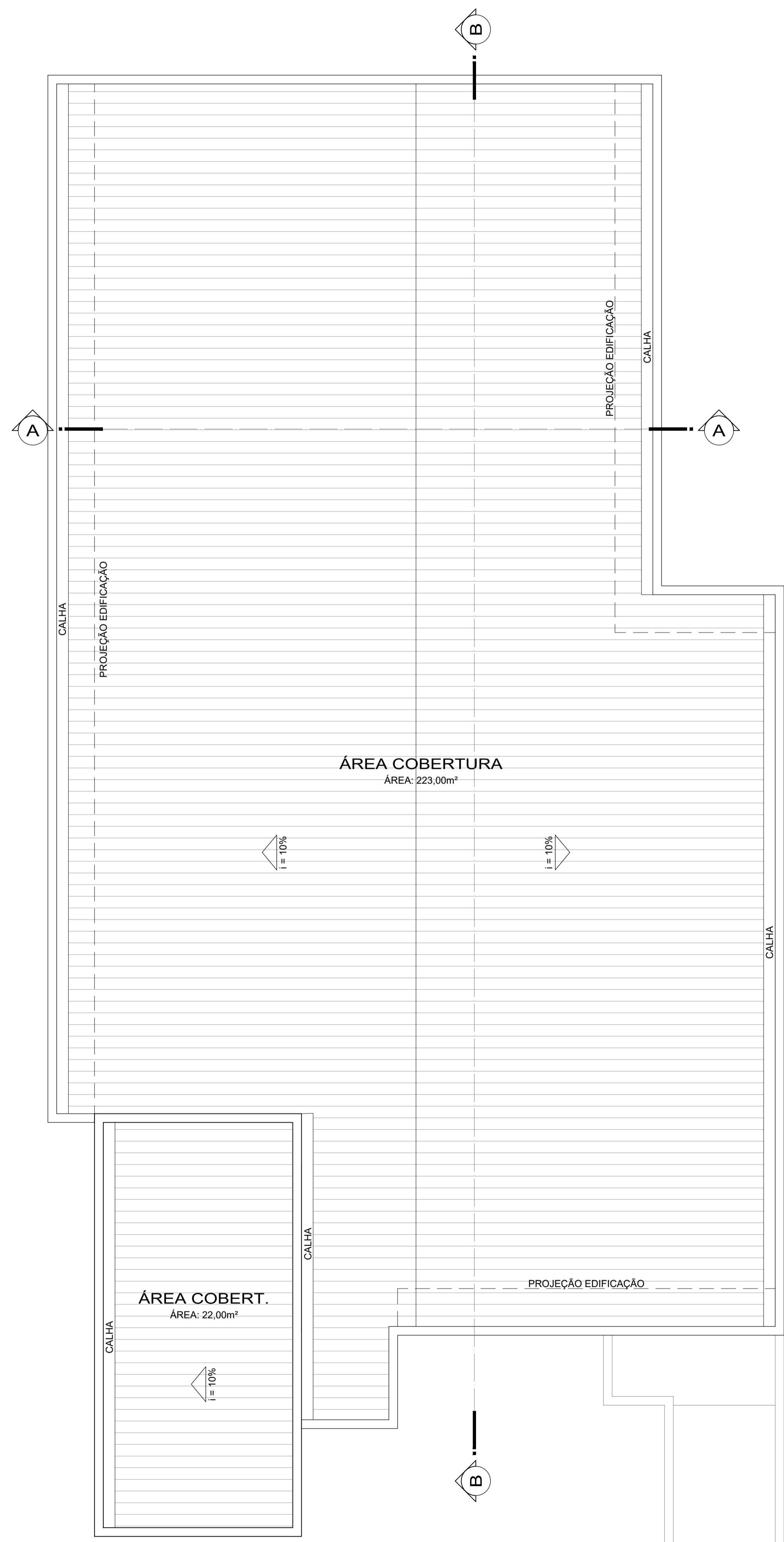
PAVTO. SUPERIOR REFORMA COBERTURA ESCALA 1/50 ÁREA TOTAL: 245,00 m²
