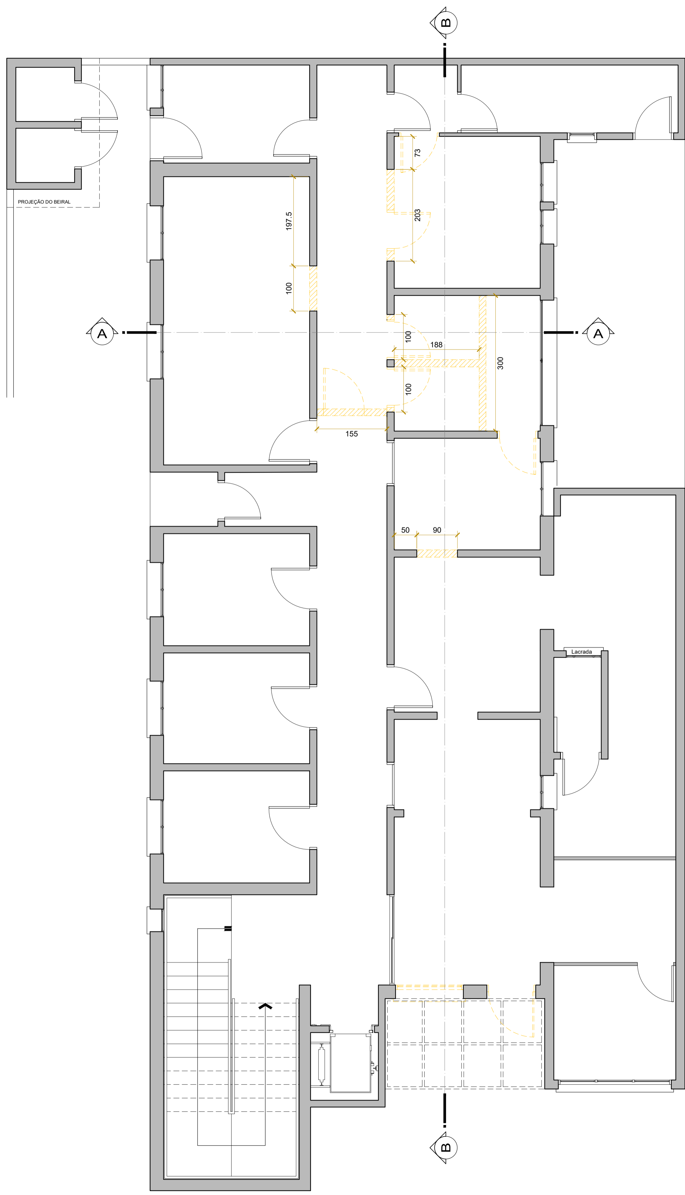
PAVTO. INFERIOR A DEMOLIR ESCALA 1/50
