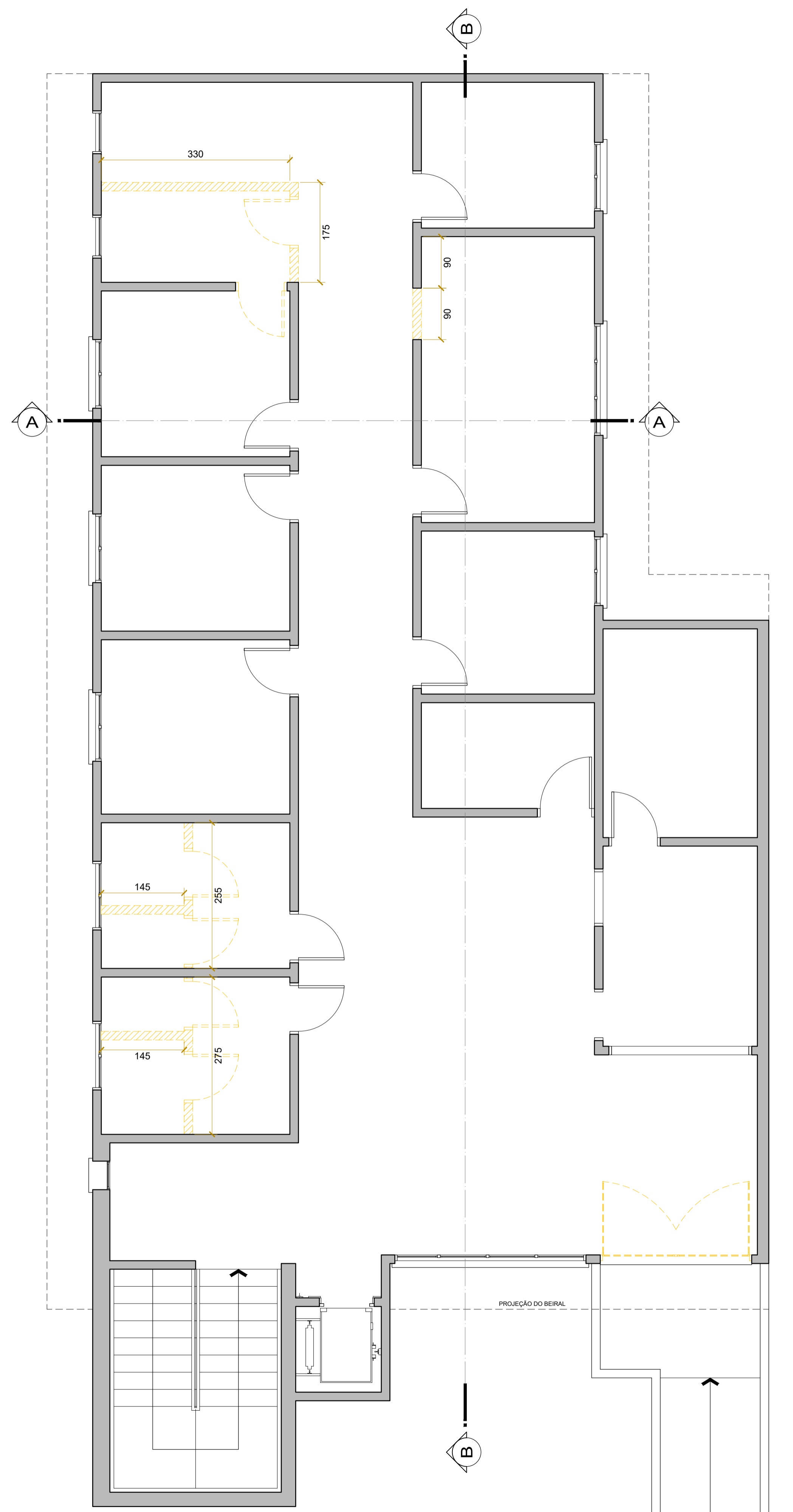
PAVTO. SUPERIOR PLANTA BAIXA ESCALA 1/50
