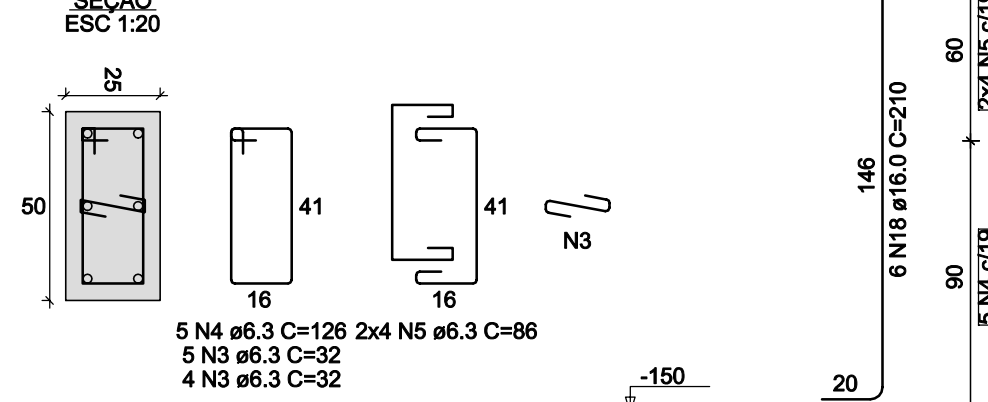
FUNDAÇÃO - L1
