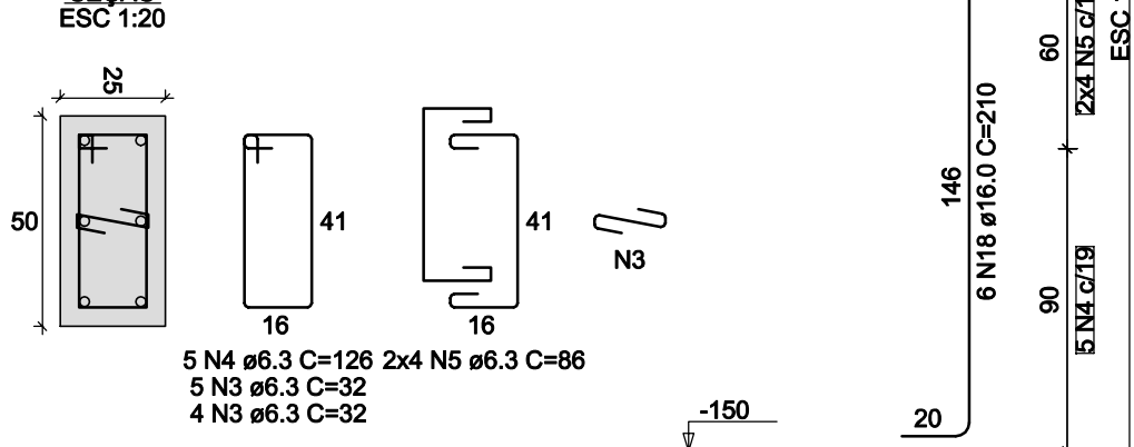
FUNDAÇÃO - L1
