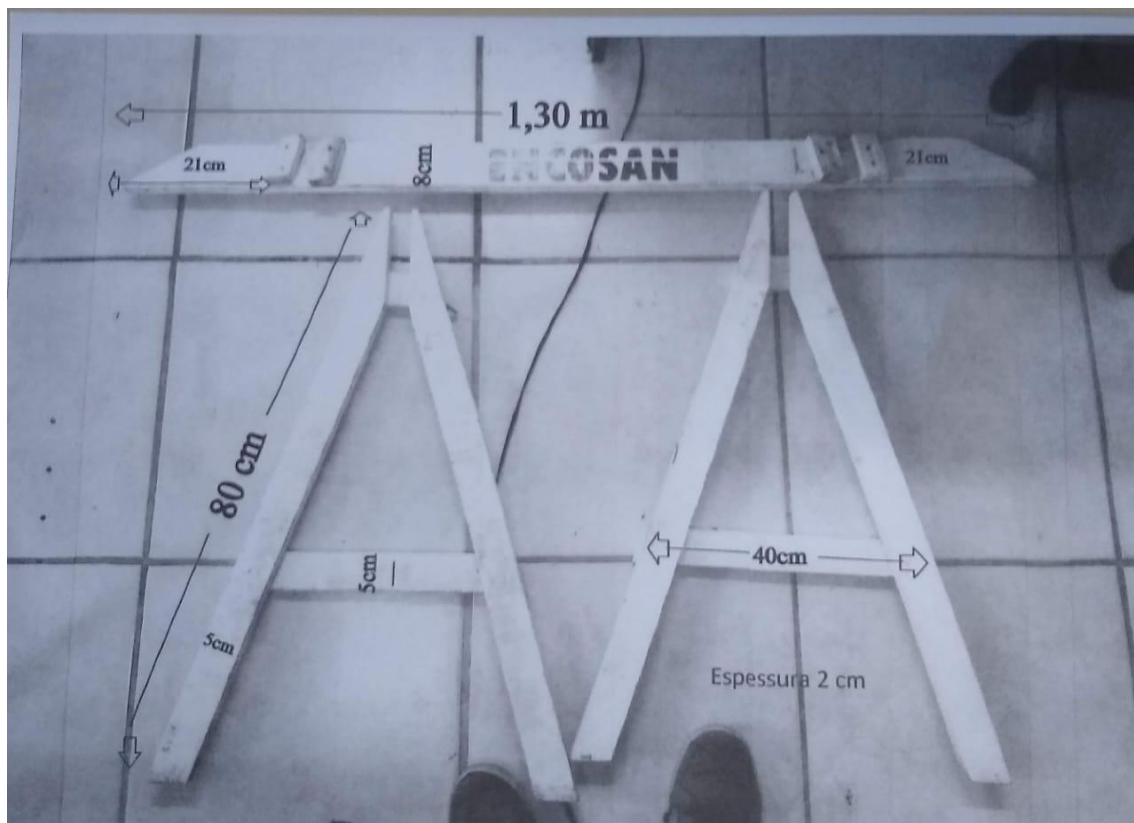
Dimensões - Imagem do cavalete de sinalização com as medidas.
