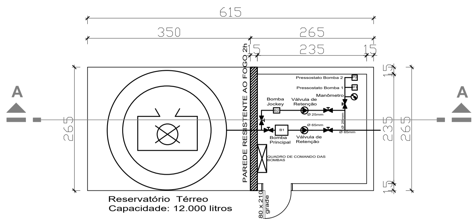
PLANTA BAIXA - CASA DE BOMBAS ESCALA 1:50
