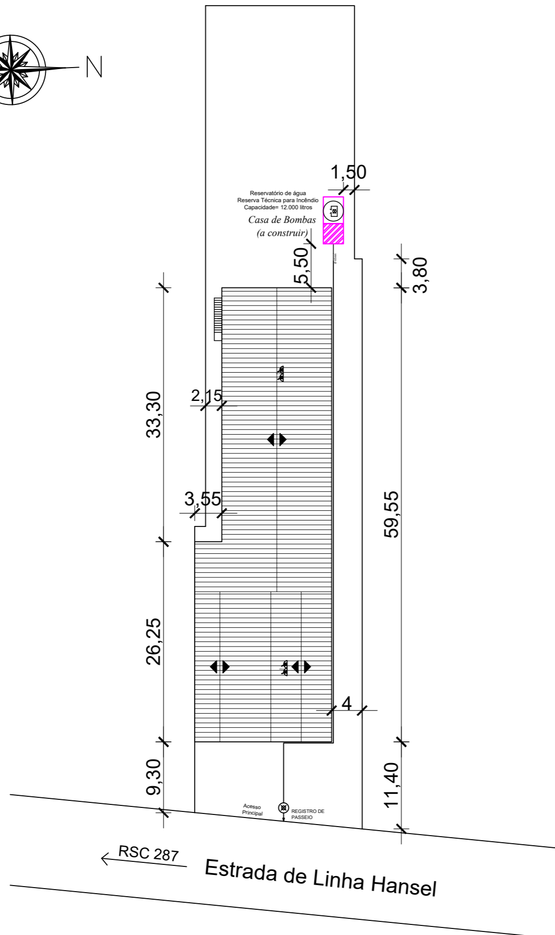
PLANTA DE IMPLANTAÇÃO ESCALA 1:1000
