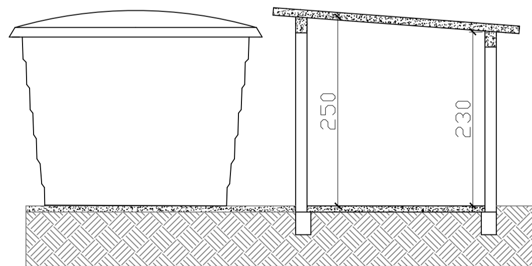
CORTE AA - CASA DE BOMBAS ESCALA 1:50
