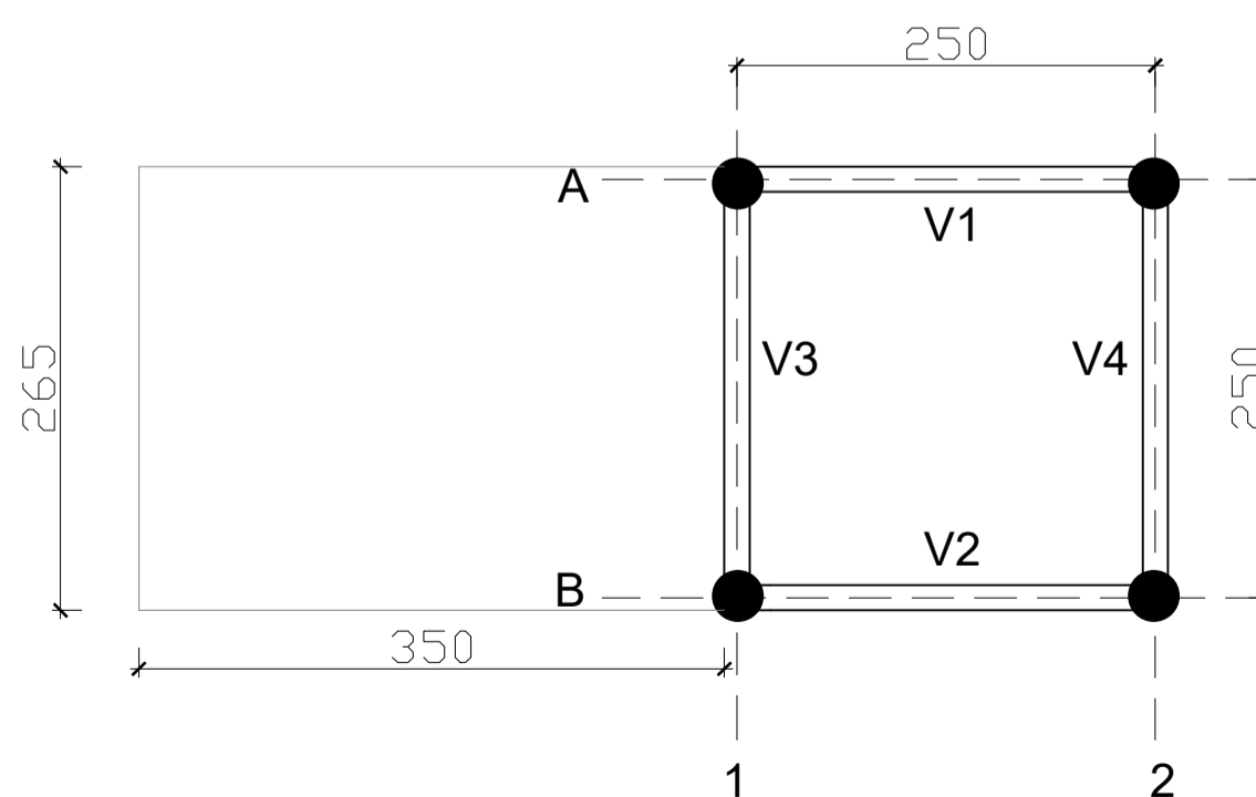
PLANTA DE LOCAÇÃO - CASA DE BOMBAS ESCALA 1:50
