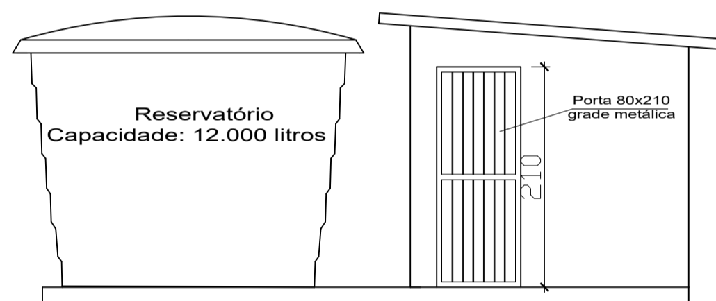
FACHADA - CASA DE BOMBAS ESCALA 1:50
