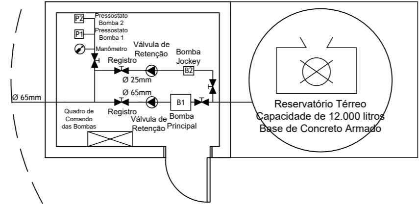
Detalhamento Casa de Bombas e Reservatório Escala 1:50
