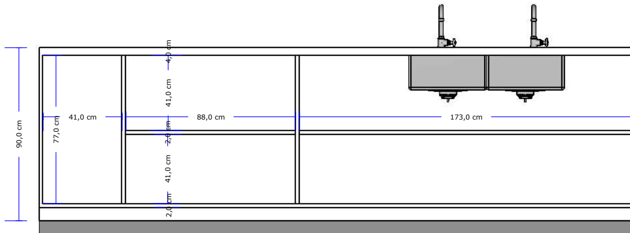
Corte - Esc:1/20
