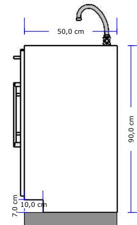
Lateral - Esc:1/20
